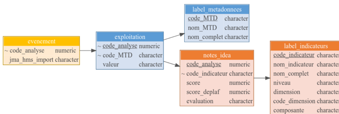
Figure 18 : Schéma des 5 tables de la base de données "IDEA_V4"
