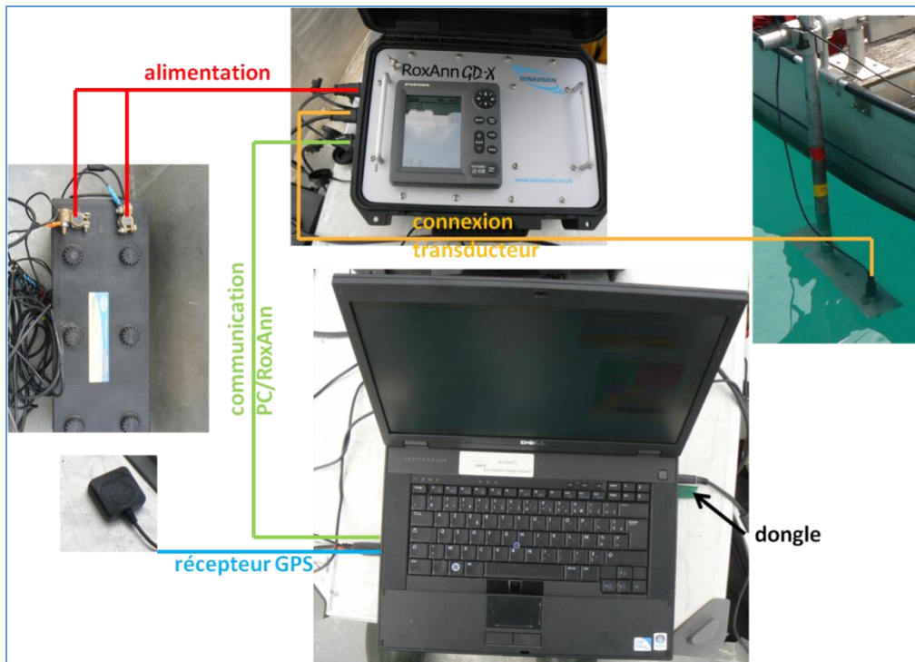
Figure 1. Matériel composant le système RoxAnn® (photos : Poulain, Argillier, et Guillard 2010).
