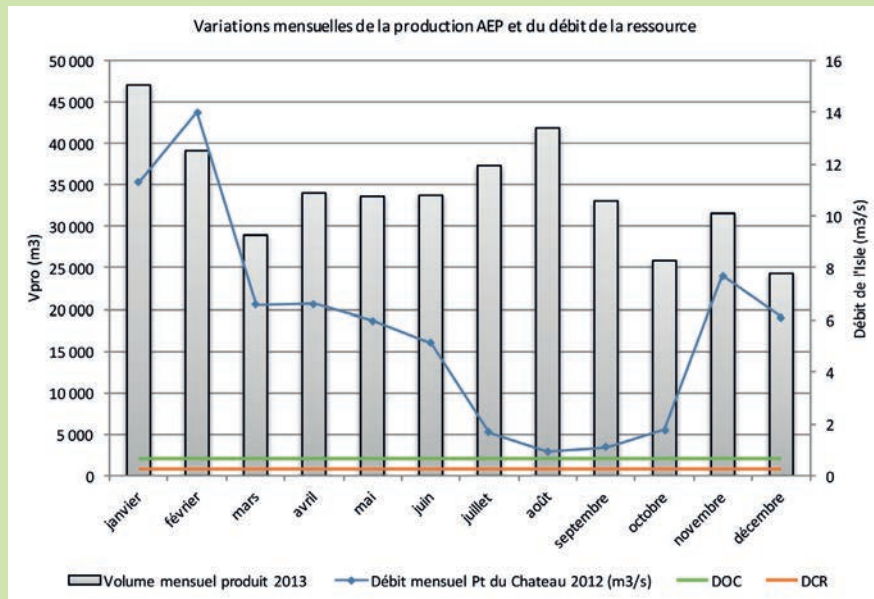
Figure 15. Mise en évidence de l'enjeu quantitatif de la ressource du syndicat de Nanthiat à l'étiage.
