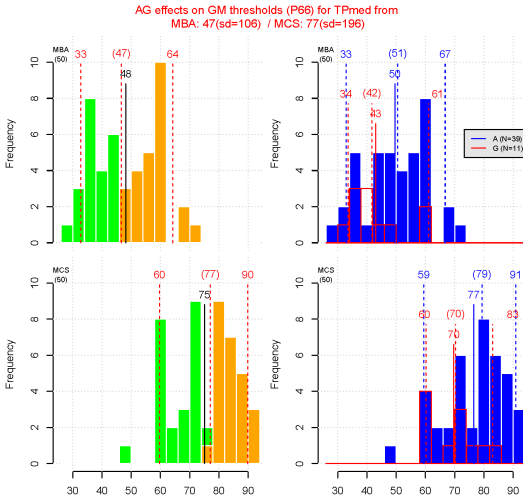
Figure 24 : Distributions des nouvelles valeurs-seuils BON/MOYEN (VS P66 ) pour la médiane des concentrations annuelles en phosphore total en zone euphotique d'après MBA (en haut) et MCS (en bas), à gauche, pour l'ensemble des plans d'eau de type étang piscicole (A) et les gravières (G) et, à droite, séparément, pour les plans d'eau de type étang piscicole (A, en bleu) et les gravières (G, en rouge).
