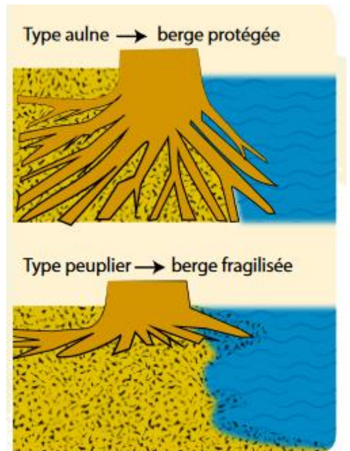
Figure 14 : Comparaison des racines de peuplier et des racines d'aulne. (Source : fédération eaux Puisaye forterre)
