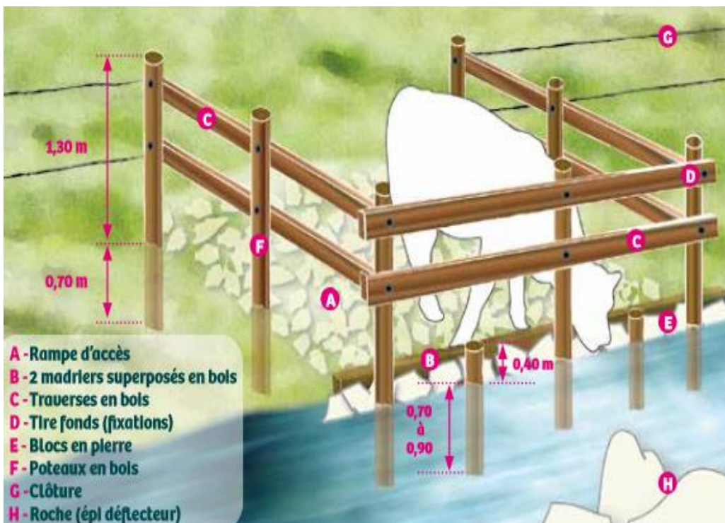
Figure 16 : Schéma d'accès aménagés de points d'abreuvement (source fédération puisaye forterre)
