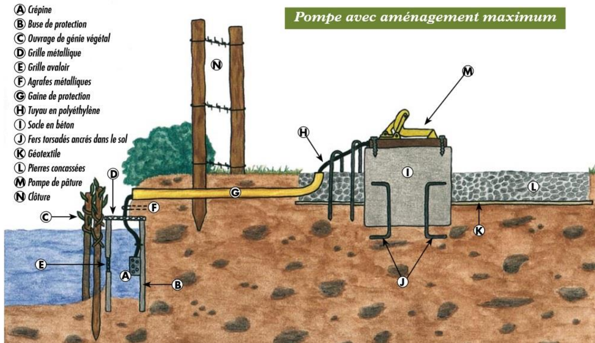
Figure 15 : Schéma d'une pompe de prairie (Source : Google image)
