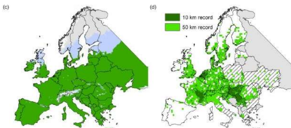
Figure 47. Stades de développement prédits pour être atteints par l'ambroisie (gauche) et présence observée de l'ambroisie (droite) en Europe (Bullock et al. 2013)
