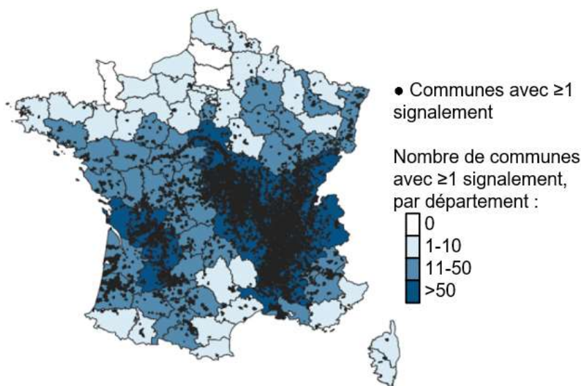
Figure 4. Carte actuelle de la répartition française de l'ambroisie d'après les données de signalements de 2010 à 2018 (Observatoire des ambrosies - FREDON France, 2019)
