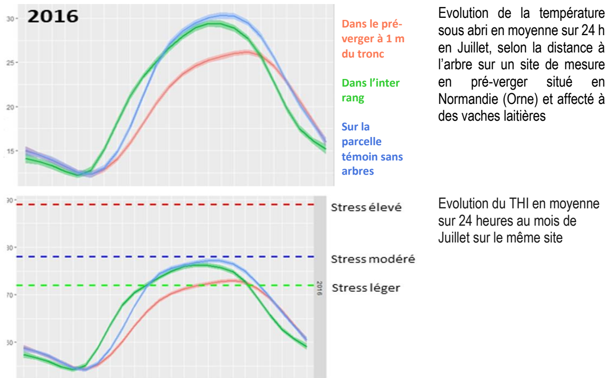
Figure 2 : Effets de l'arbre sur le ressenti de l'animal, approché par le calcul du THI
