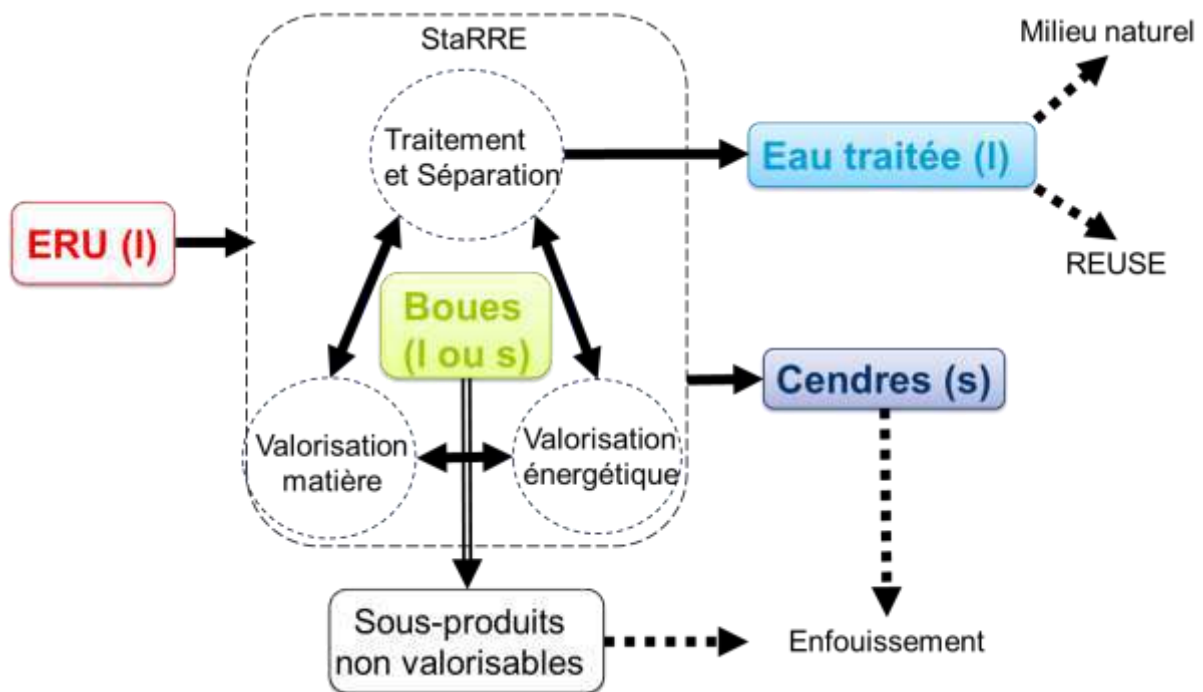
Figure 6 : Matrices (cadres en trait pleins) et flux principaux des itinéraires technologiques d'assainissement
