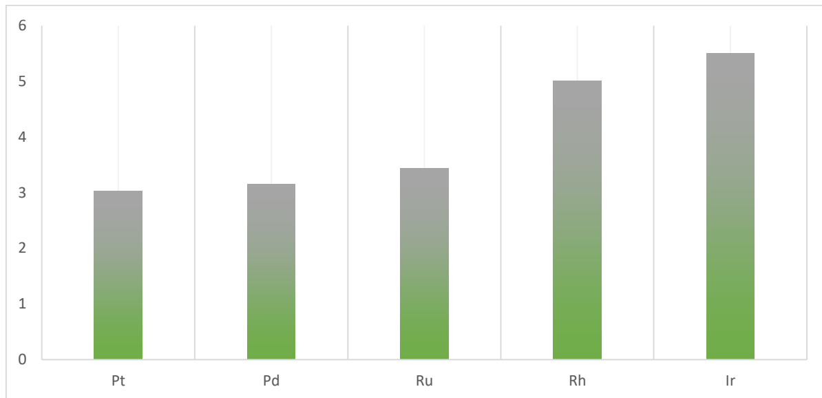
Figure 24 : Facteur de concentration des métaux du passage de la matrice boues à la matrice cendres – métaux rangés du plus au moins concentré. (Jackson et al., 2010)
