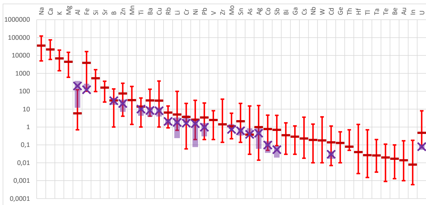
Figure 19 : Flux journalier arrivant en STEP exprimé en mg/EH/j, les données suisses (Vriens et al., 2017) en rouge et les données du projet Ampères (Choubert et al., 2011) en violet
