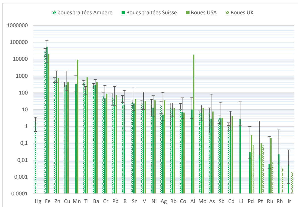
Figure 22 : Teneurs en métal dans les boues en \text{mg.kg}^{-1}\text{MS} . Moyenne et écart-type du projet Ampere (Choubert et al., 2011) ; minimum, médiane, maximum du projet Suisse (Vriens et al., 2017) ; médiane des échantillons composites du projet USA (Westerhoff et al., 2015) et médiane du projet anglais (Jackson et al., 2010)
