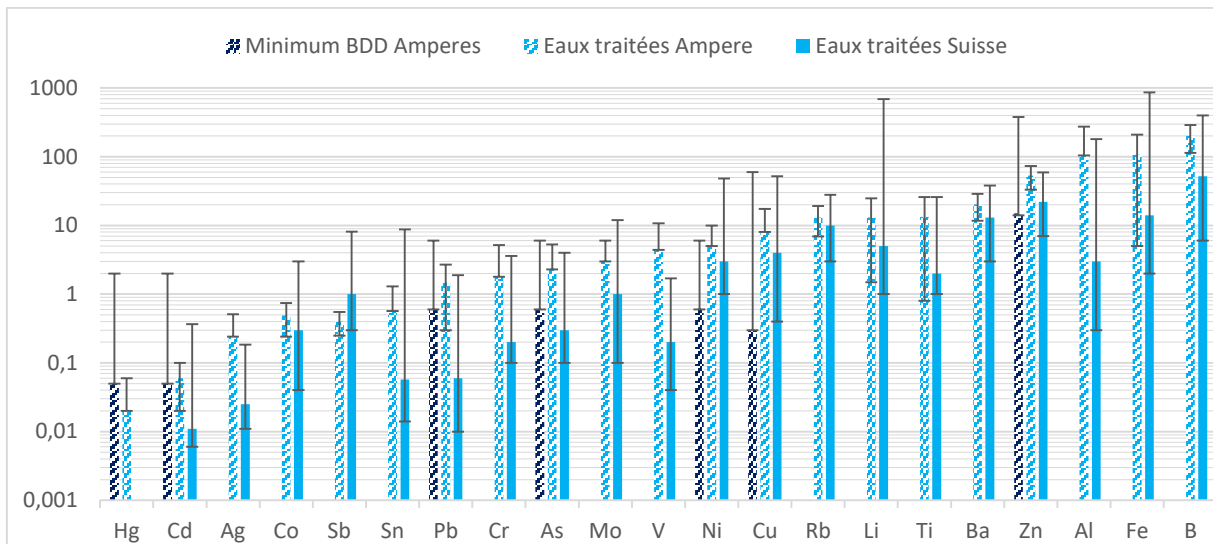
Figure 20 : Plages de concentration des métaux dans les eaux traitées. Données du projet Ampere (moyenne et écart type) et de l'étude nationale Suisse (médiane et extremum)
