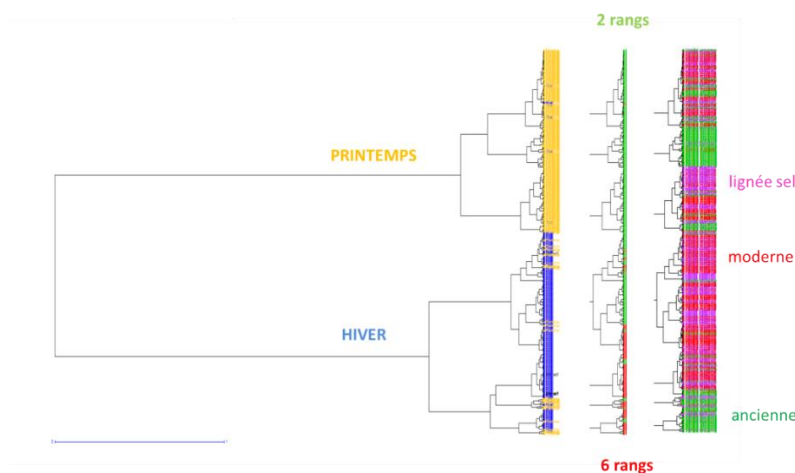
Figure 3 : Structuration génétique au sein de la collection nationale d'orge
