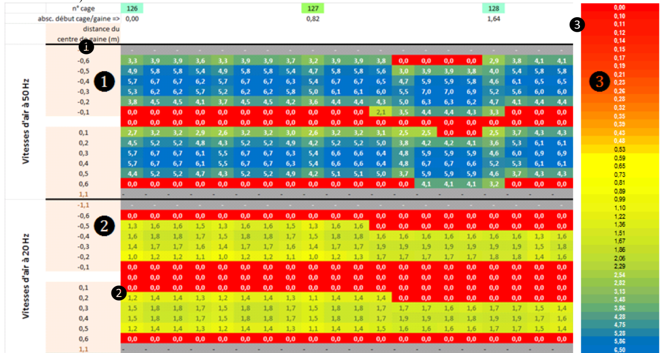
Figure 2. : exemple de sorties couleur selon les vitesses d'air calculées dans les logements au niveau 0 (fond de la loge ; absc.=distance au ventilateur en m) sur le visuel du schéma de sortie – ① = à puissance maxi du ventilateur – ② = à puissance mini du ventilateur - ③ échelle des couleurs utilisées selon les vitesses d'air calculées (m/s) ; les variations spatiales s'expliquent notamment par le choix de 2 lignes de trous et la présence des séparations de logements ; les différences entre les cartes ① et ② s'expliquent par la répartition des pressions dans la gaine en fonction du perçage et du ventilateur)
