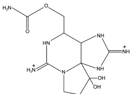
Figure 5 : structure chimique de la saxitoxine
