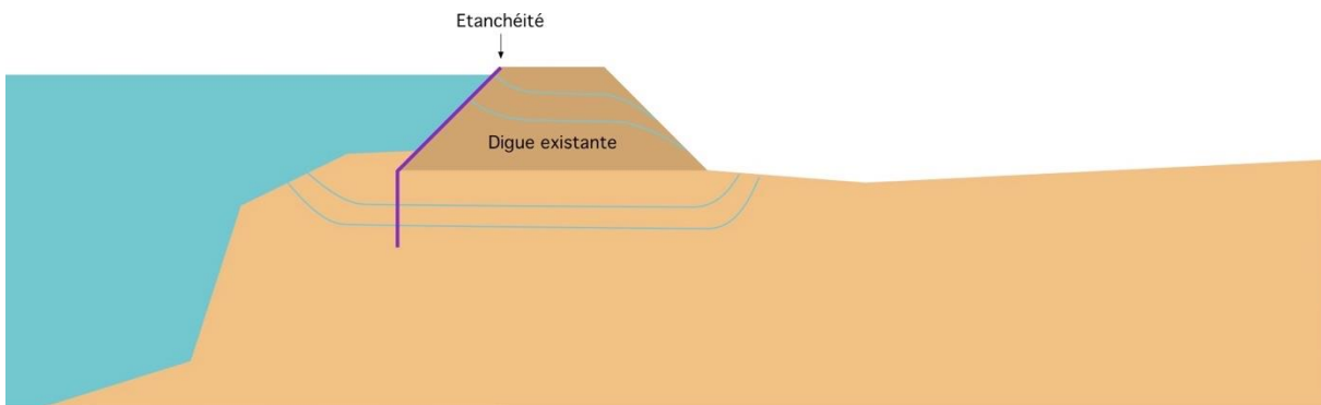
Figure 3.2 : Étanchéité par masque amont pour la digue et la fondation. NB : les courbes correspondent aux lignes d'écoulement (et donc les chemins potentiels d'érosion) avant la mise en place des étanchéités (Source : R. Tourment)
