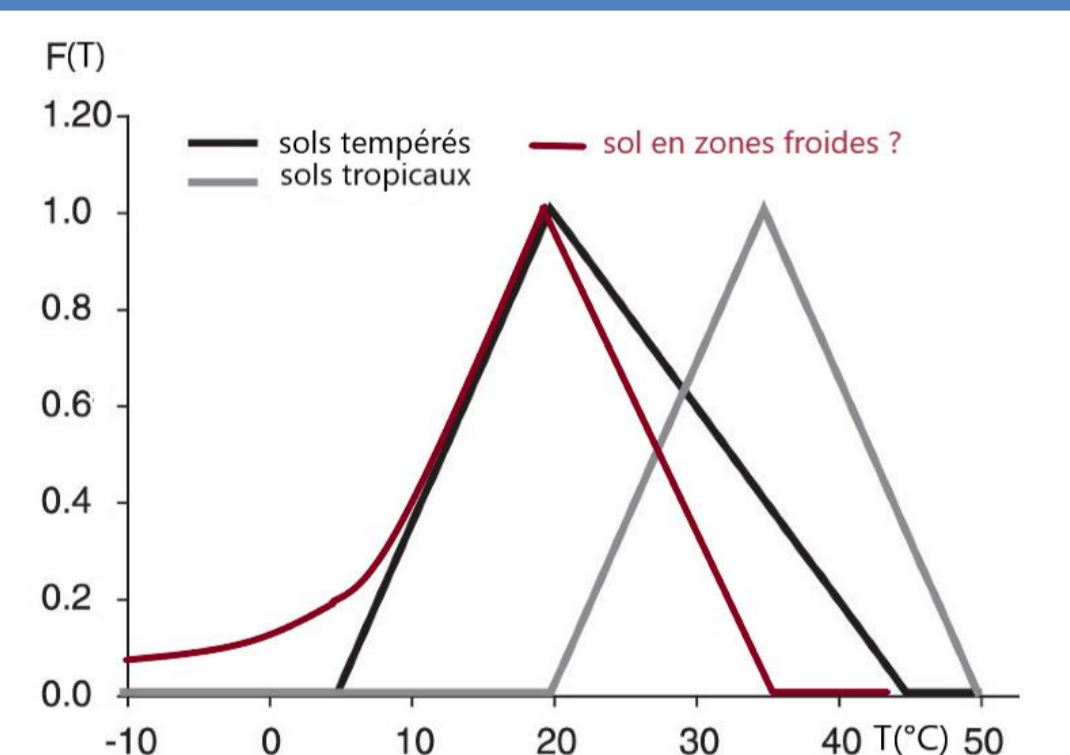
Fig. 4 : Effet de la T° sur la nitrification
