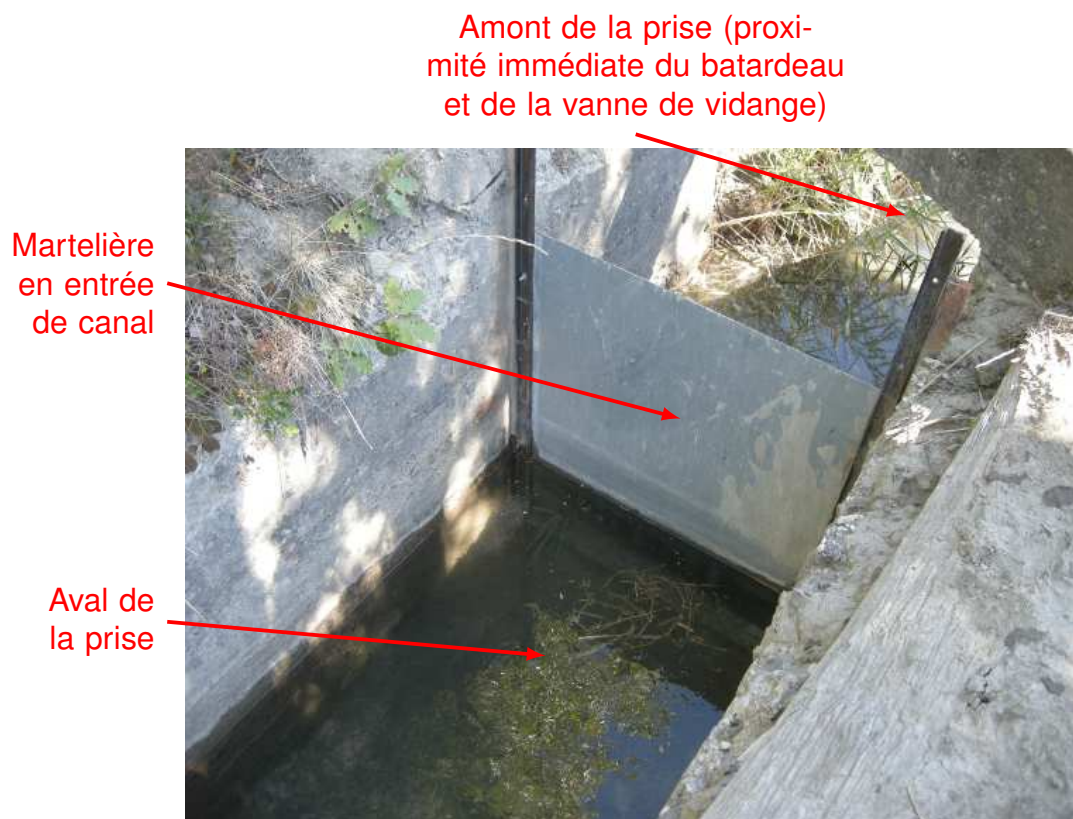
FIGURE 4.6 – Photo de la prise d'eau Canal du Moulin : vanne à l'entrée du canal
