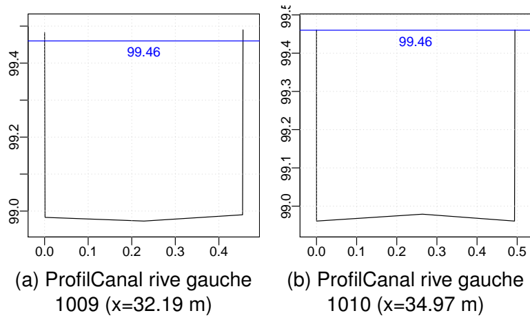
FIGURE 11.90 – Profils en travers (Canal rive gauche)
