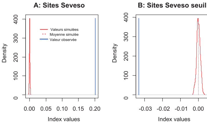
Fig. 2 Test de significativité (permutations de Monte Carlo) de la centralisation environnementale
