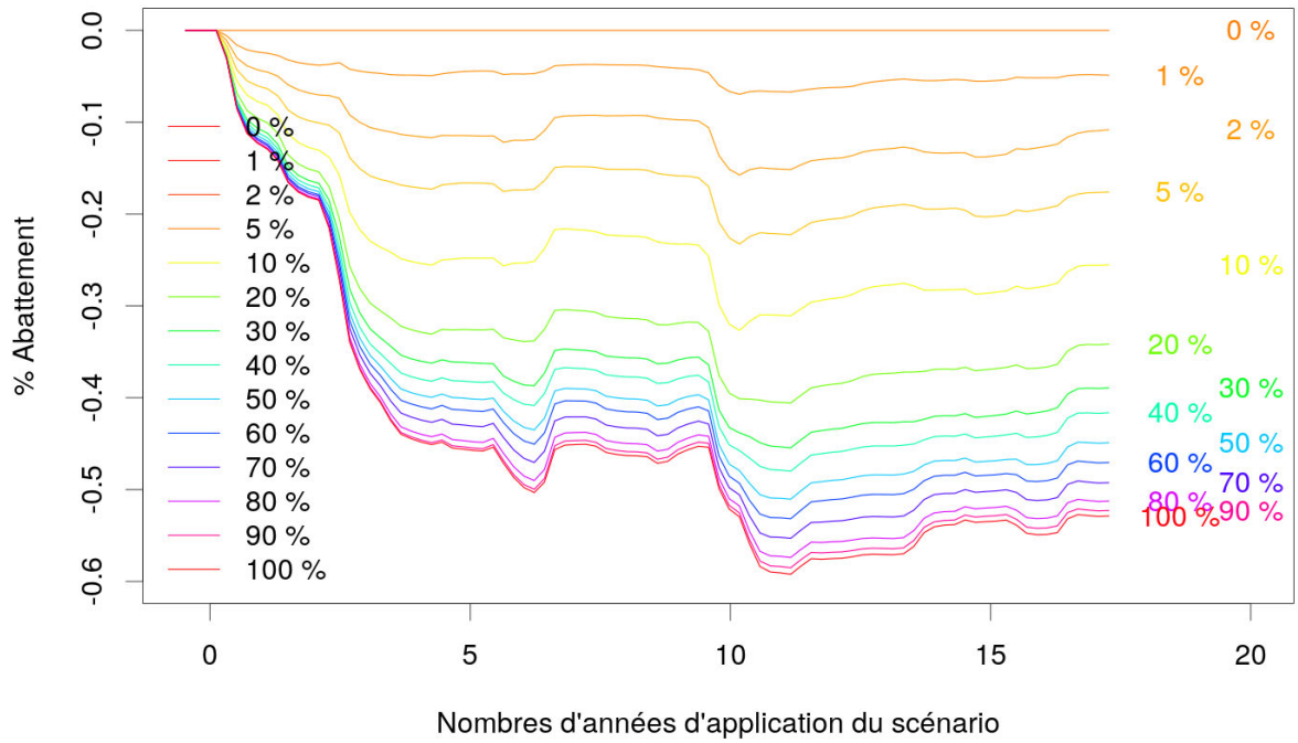
Figure 21: Scénario BSC, Y finiac, Abattement estival en fonction de la durée d'application, pour plusieurs valeurs de surfaces modifiées (0-100%). Pour l'échelle d'abattement, -0,3 correspond à un abattement de 30 % du flux de référence ou, autrement dit, le flux du scénario correspond à 70 % du flux de référence.
