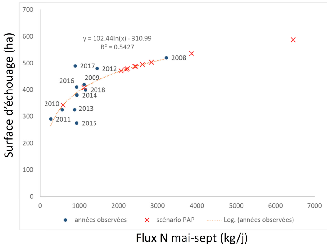
Figure 8: Surface d'échouage des algues en fonctions des flux d'azote estivaux (Les années dites observées sont issues de simulations MARS-Ulves à partir des séries de référence simulées par TNT2).
