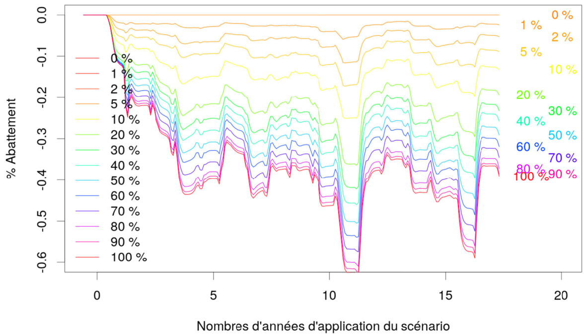
Figure 5: Scénario BSC Y ffiniac. Abattement annuel en fonction de la durée d'application, pour plusieurs valeurs de surfaces modifiées (0-100%). Pour l'échelle d'abattement, -0,3 correspond à un abattement de 30 % du flux de référence ou, autrement dit, le flux du scénario correspond à 70 % du flux de référence.
