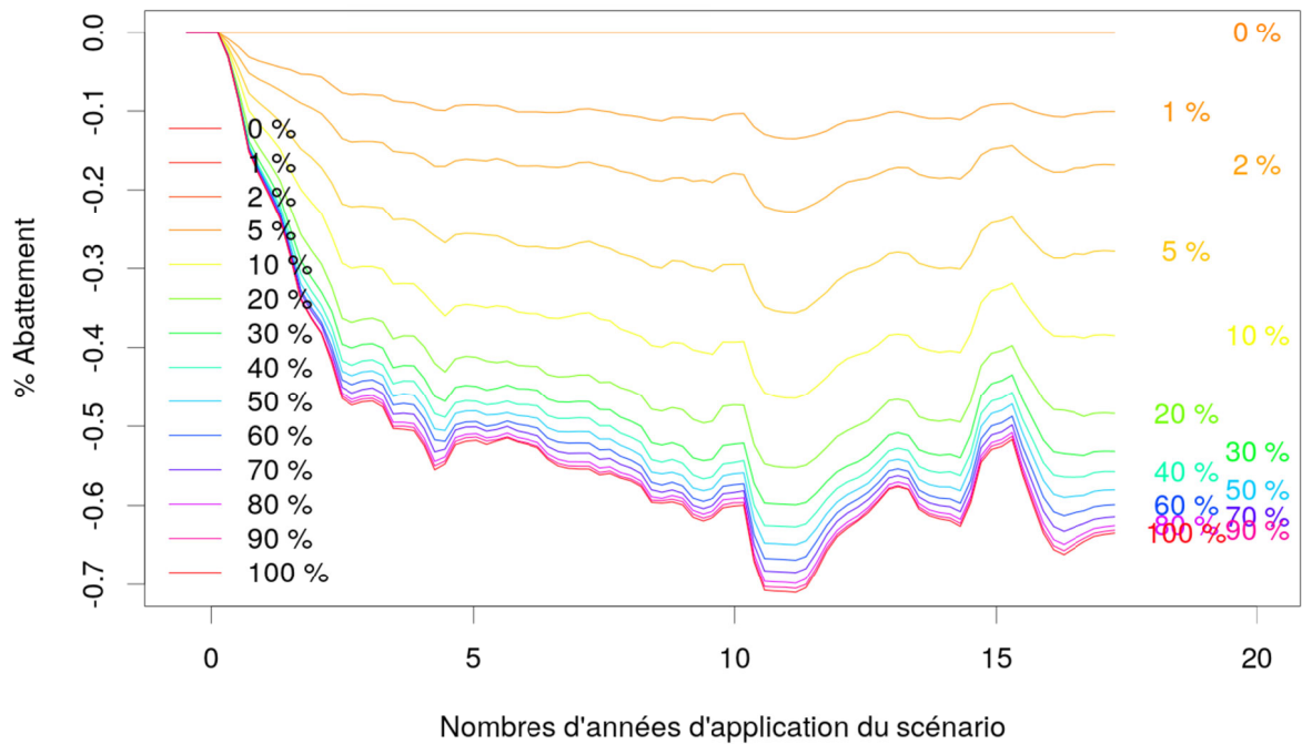
Figure 2: Scénario BSC, ensemble des trois bassins versants, Abattement pour la saison estivale (mai-sept.) en fonction de la durée d'application, pour plusieurs valeurs de surfaces modifiées (0-100%). Pour l'échelle d'abattement, -0,3 correspond à un abattement de 30 % du flux de référence ou, autrement dit, le flux du scénario correspond à 70 % du flux de référence.
