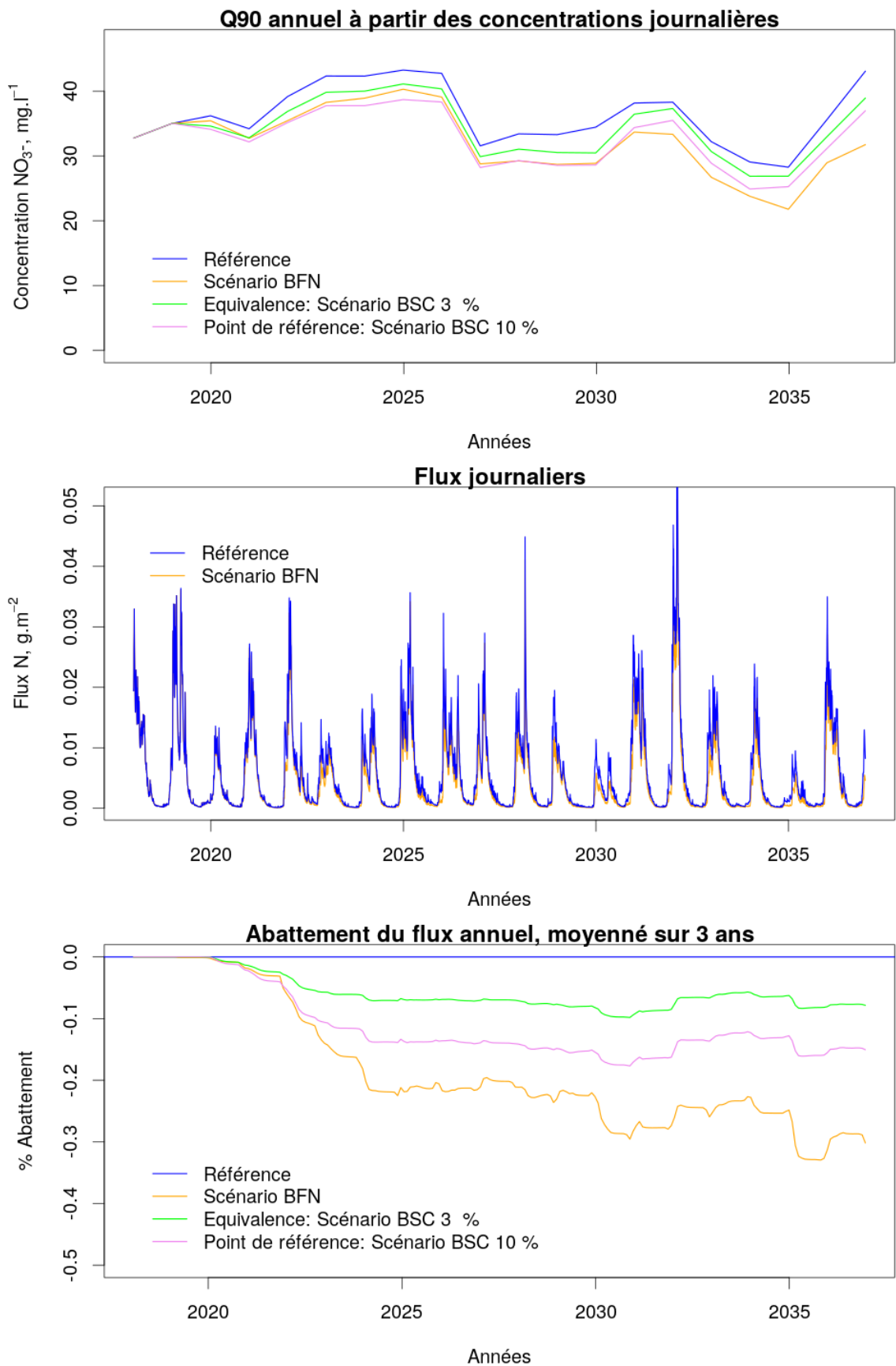
Figure 12: Scénario BFN sur Y ffiniac. Quantile 90 des concentrations en nitrate, flux d'azote et abatement annuel (tendance à 3 ans). Comparaison avec un scénario BSC présentant un abatement après 15 ans équivalent, et avec BSC 10 % pour référence.
