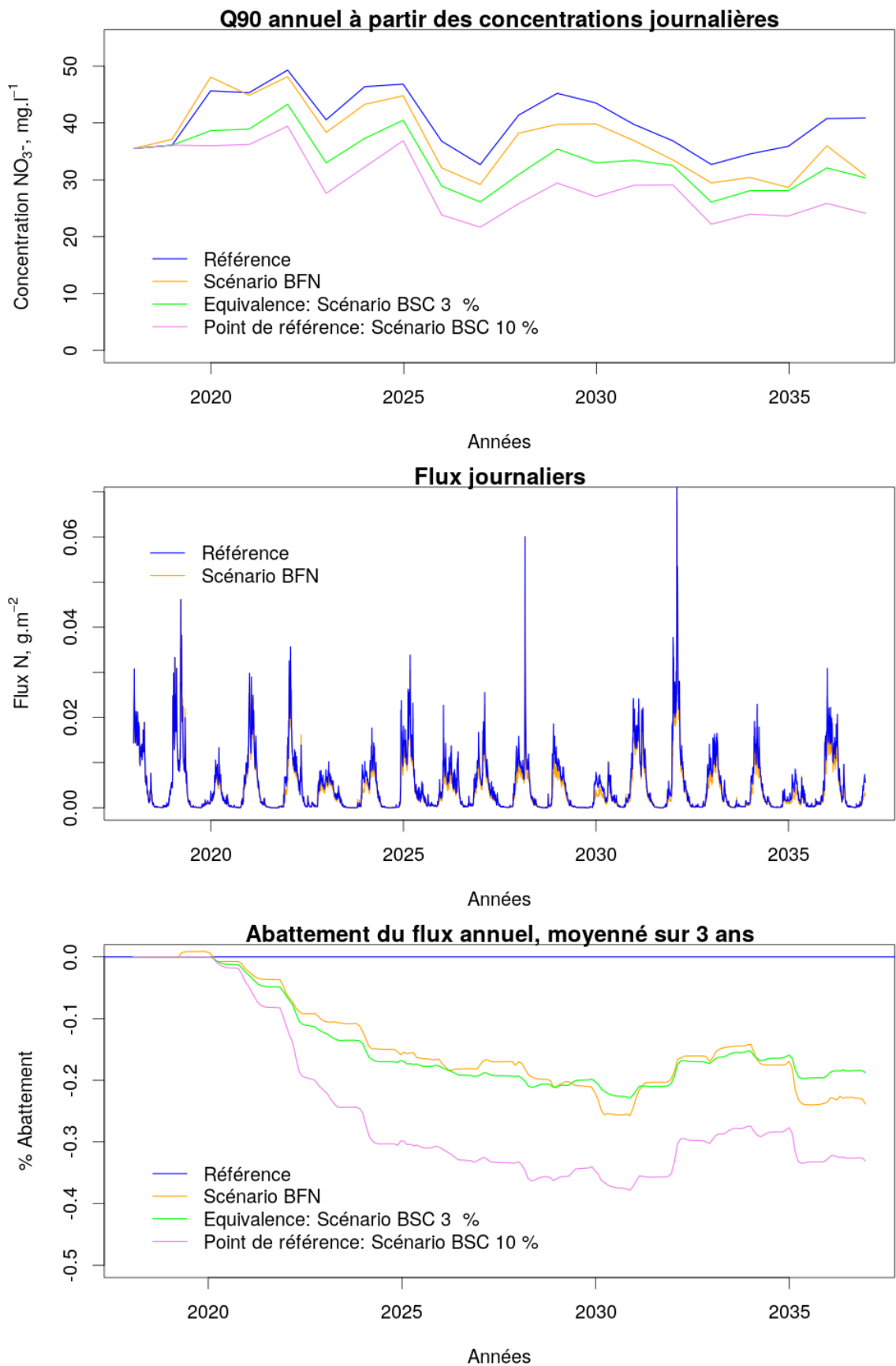
Figure 10: Scénario BFN sur le Gouessant. Quantile 90 des concentrations en nitrate, flux d'azote et abattement annuel (tendance à 3 ans). Comparaison avec un scénario BSC présentant un abattement après 15 ans équivalent, et avec BSC 10 % pour référence.
