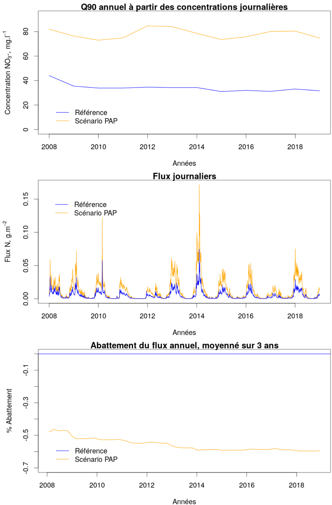
Figure 7: Scénario PAP sur les trois bassins versants. Quantile 90 des concentrations en nitrate, flux d'azote et abattement annuel (tendance à 3 ans)
