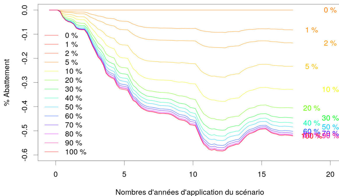
Figure 18: Scénario BSC, Gouet, Abattement estival en fonction de la durée d'application, pour plusieurs valeurs de surfaces modifiées (0-100%). Pour l'échelle d'abattement, -0,3 correspond à un abattement de 30 % du flux de référence ou, autrement dit, le flux du scénario correspond à 70 % du flux de référence.
