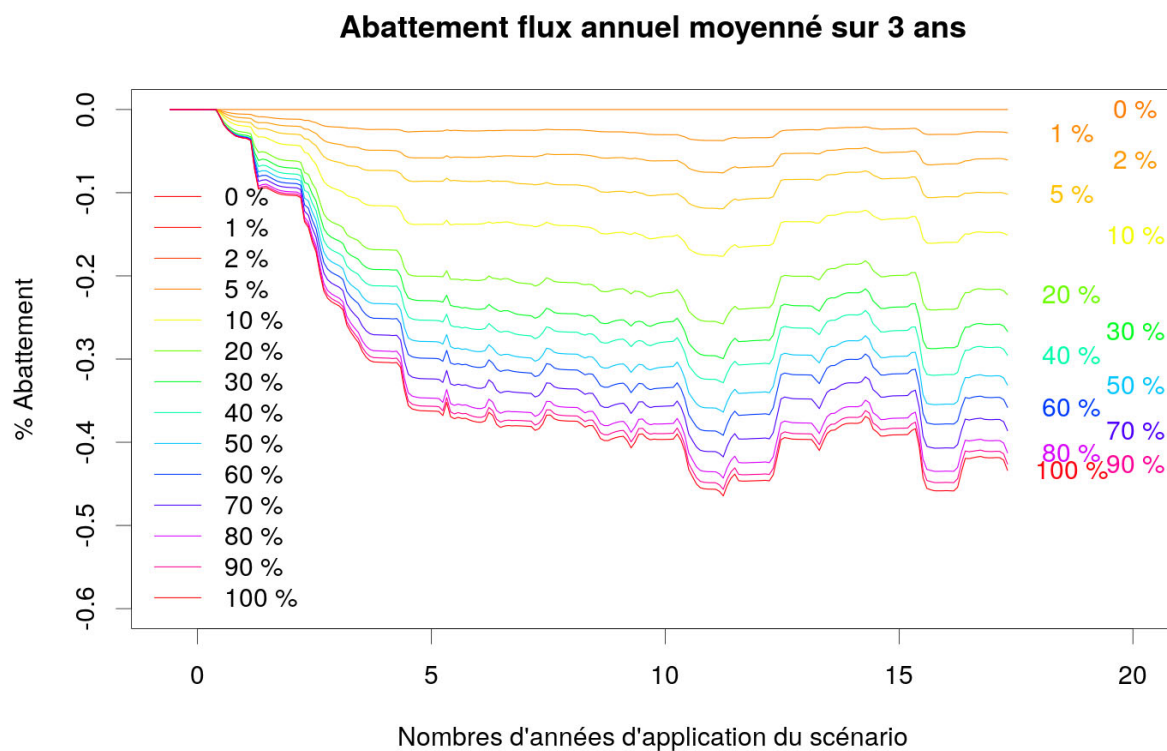
Figure 20: Scénario BSC, Y ffiniac, Abatement annuel en fonction de la durée d'application, pour plusieurs valeurs de surfaces modifiées (0-100%). Pour l'échelle d'abattement, -0,3 correspond à un abattement de 30 % du flux de référence ou, autrement dit, le flux du scénario correspond à 70 % du flux de référence.
