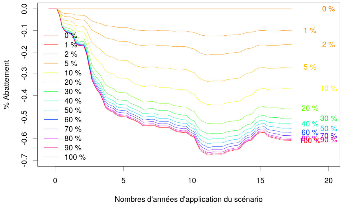
Figure 4: Scénario BSC, ensemble des trois bassins versants, Abattement pour la saison estivale (mai-sept.) en fonction de la durée d'application, pour plusieurs valeurs de surfaces modifiées (0-100%). Pour l'échelle d'abattement, -0,3 correspond à un abattement de 30 % du flux de référence ou, autrement dit, le flux du scénario correspond à 70 % du flux de référence.
