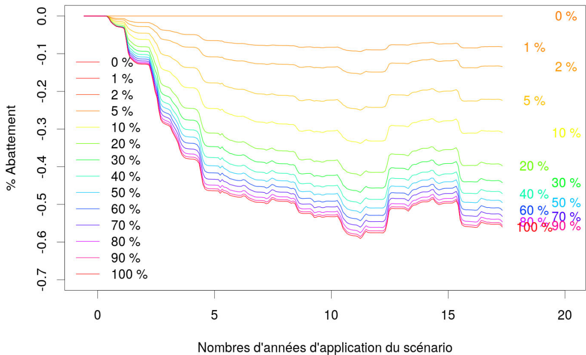
Figure 3: Scénario BSC, ensemble des trois bassins versants, Abattement annuel en fonction de la durée d'application, pour plusieurs valeurs de surfaces modifiées (0-100%). Pour l'échelle d'abattement, -0,3 correspond à un abattement de 30 % du flux de référence ou, autrement dit, le flux du scénario correspond à 70 % du flux de référence.
