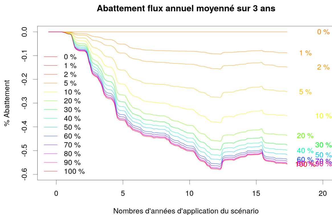
Figure 17: Scénario BSC, Gouet, Abattement annuel en fonction de la durée d'application, pour plusieurs valeurs de surfaces modifiées (0-100%). Pour l'échelle d'abattement, -0,3 correspond à un abattement de 30 % du flux de référence ou, autrement dit, le flux du scénario correspond à 70 % du flux de référence.
