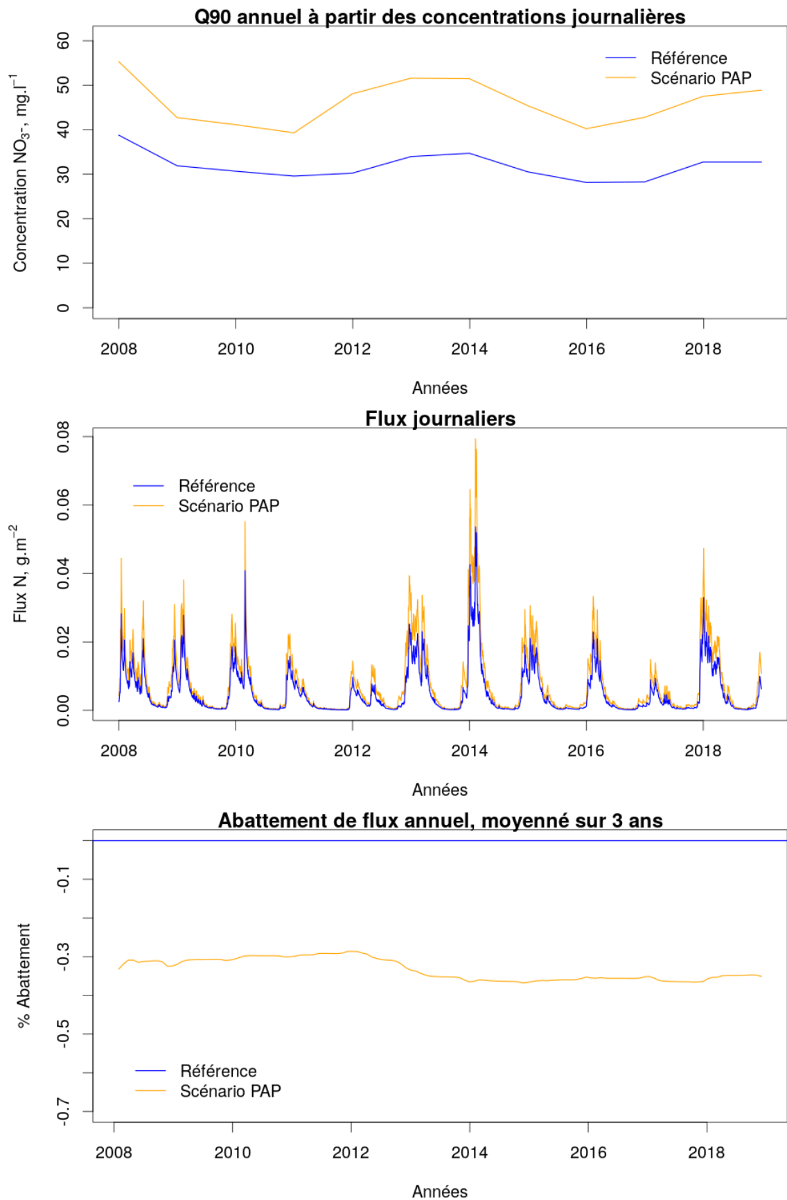
Figure 22: Scénario PAP, Y ffiniac. Quantile 90 des concentrations en nitrate, flux d'azote et abattement annuel (tendance à 3 ans)
