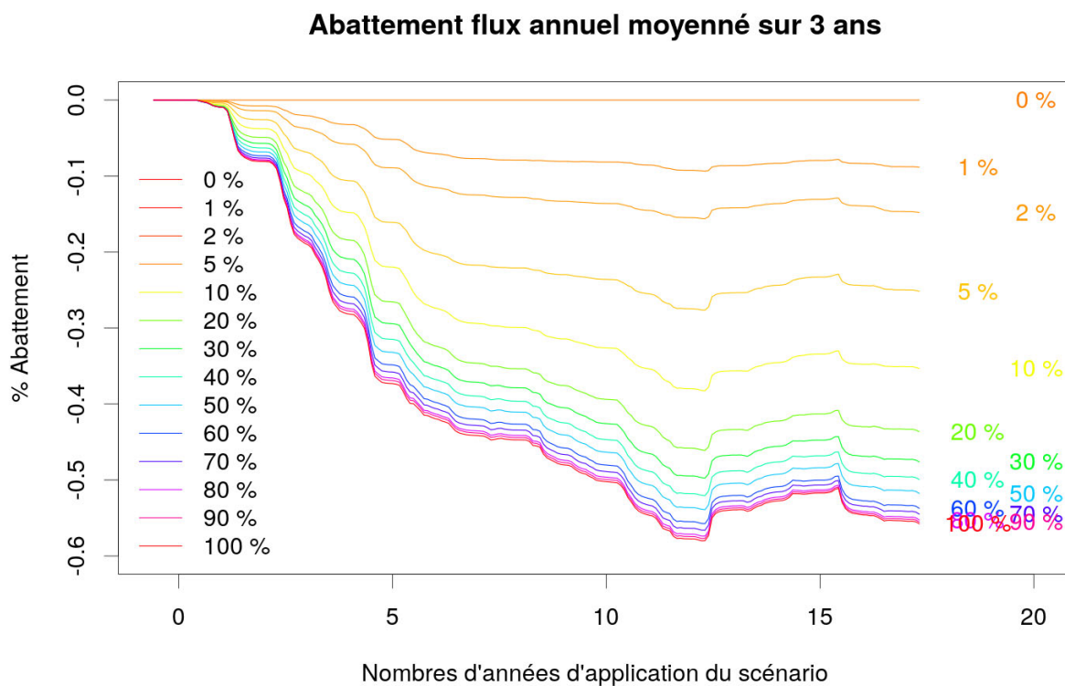
Figure 17: Scénario BSC, Gouet, Abatement annuel en fonction de la durée d'application, pour plusieurs valeurs de surfaces modifiées (0-100%). Pour l'échelle d'abattement, -0,3 correspond à un abattement de 30 % du flux de référence ou, autrement dit, le flux du scénario correspond à 70 % du flux de référence.
