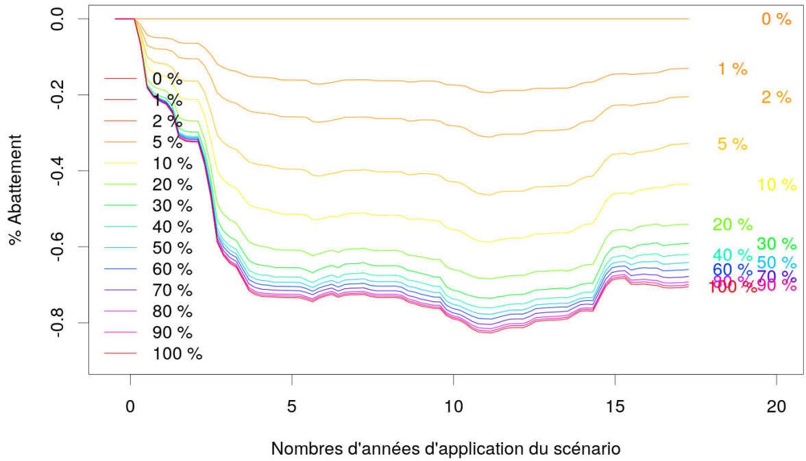
Figure 15: Scénario BSC, Guessant, Abattement estival en fonction de la durée d'application, pour plusieurs valeurs de surfaces modifiées (0-100%). Pour l'échelle d'abattement, -0,3 correspond à un abattement de 30 % du flux de référence ou, autrement dit, le flux du scénario correspond à 70 % du flux de référence.
