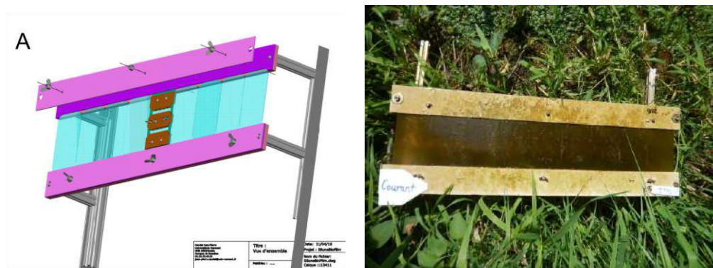
Figure 17. Système de fixation des lames pour les stations lotiques (à gauche) et lames dans leurs supports après colonisation (à droite).
