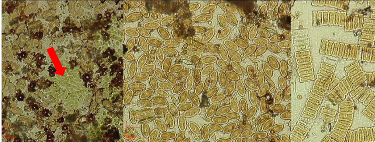
Fig. 4 : quelques photos du biofilm (periphyton) observé dans les affluents. La flèche rouge montre une algue verte, tandis que les autres sont différentes espèces de diatomées benthiques.
