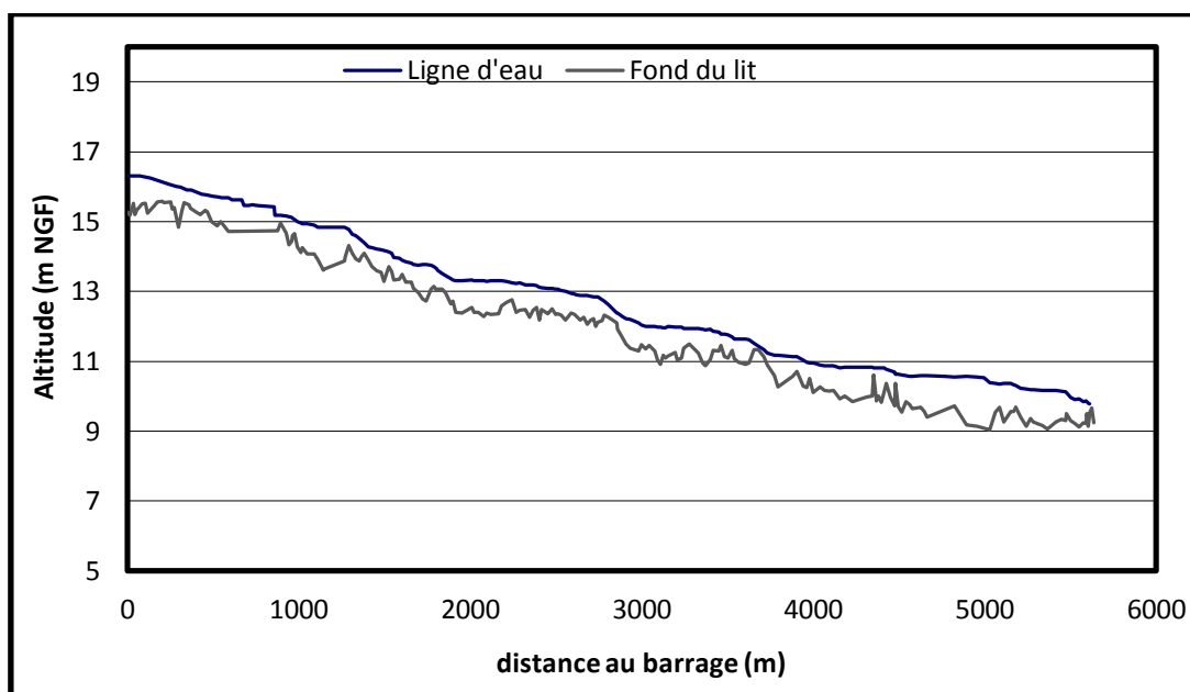
Figure 27 : profil en long de la Sélune en aval du barrage de la Roche qui Boit (Fond du lit et ligne d'eau)
