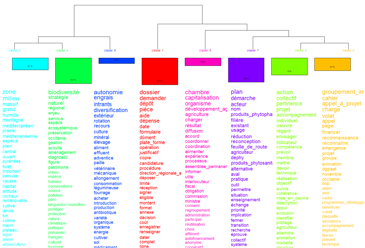
Figure 5 : Dendrogramme issu de l'analyse textuelle des 23 textes régionaux
