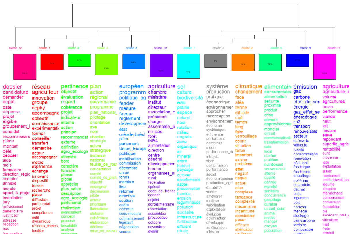
Figure 2 : Dendrogramme issu de l'analyse textuelle des 163 textes du corpus
