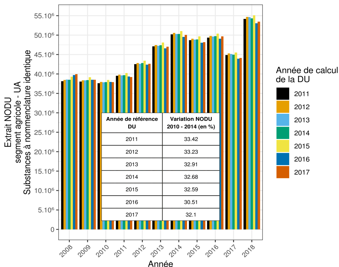
Figure 1.1.2 : NODU du segment agricole-UA calculés au moyen des différents DU calculées entre 2011 et 2017 et réropolés sur toutes les années. NODU du segment agricole - UA calculés au moyen des différents DU calculées entre 2011 et 2017 et réropolées sur toutes les années.
