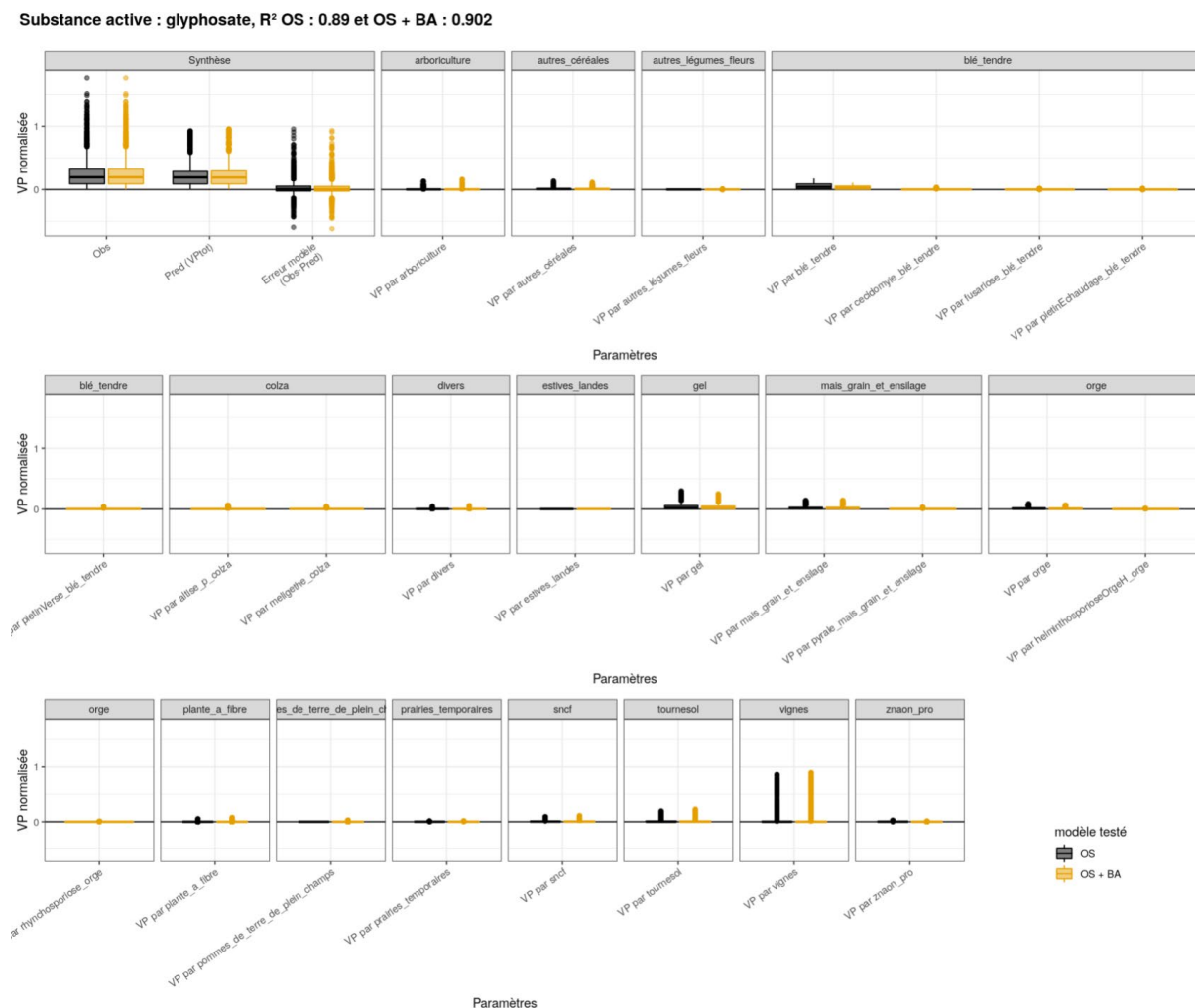
Fig 2.4.12 : Variations Prédites normalisées (VP/surface totale modélisée PRA) en glyphosate pour chaque année et chaque PRA par les occupations du sol (OS) et les bioagresseurs (BA) sélectionnés, ainsi que l'erreur associée au modèle Lasso réalisé et au modèle nul selon le type de modèle réalisé : modèle avec les occupations du sol seul (OS) ou incluant la pression en bioagresseurs (OS + BA). Les valeurs de R^2_{\text{ajusté}} des différents modèles sont présentées dans le titre.
