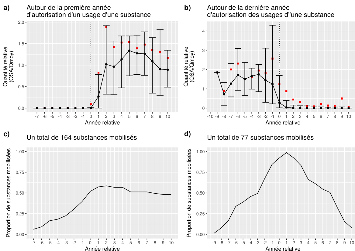
Figure 2.1.2 : Evolution des quantités de substances actives, exprimées en quantité relative ( QR_{SA} = Q_{SA} / Q_{SA \text{ moyenne}} ), par rapport a) la première année d'autorisation d'un usage et b) l'année où tous les usages sont interdits. Les années sont exprimées en Année relative (Année relative = Année réelle - Année pivot). Les points, la courbe et les écart-types noirs représentent la QR_{SA} médiane avec les quantiles à 0.25 et 0.75. Les carrés rouges représentent les moyennes des QR_{SA} . c) et d) représentent les proportions des substances mobilisées pour le calcul des statistiques par année relative pour a) et b), respectivement.
