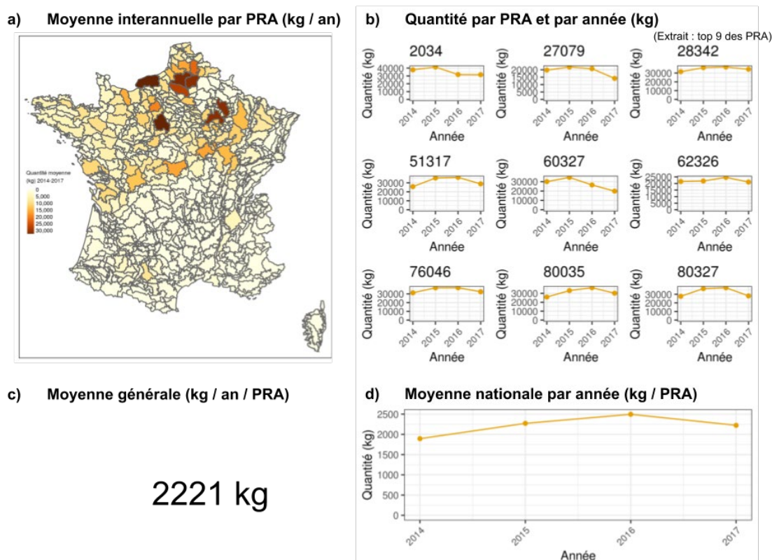
Fig. 2.4.5 : Variabilité temporelle et spatiale des quantités vendues de chlorothalonil dans la BNV-d Registre segment agricole - UA, hors AMM stockage, entre 2014 et 2017 : a) moyenne interannuelle des quantités vendues dans chaque PRA, b) Evolution temporelle des quantités vendues dans les 9 PRA les plus importantes en termes de quantités totales vendues (codes des PRA renseignés dans les titres), c) moyenne des quantités sur la période et l'ensemble des PRA et d) moyenne nationale des quantités vendues chaque année.
