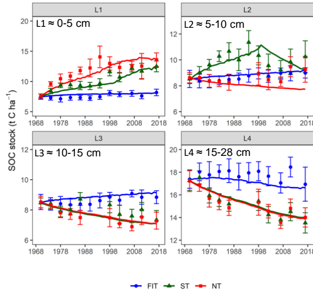
b) AMGv3
