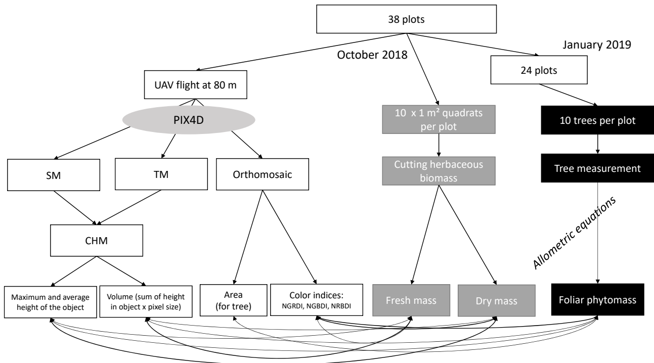
Figure 1: Graphic representation of the methodology used to assess grass and foliar phytomass with UAV in Sahelian savanna; SM: surface model; TM: terrain model; CHM: canopy height model; NRB DI = normalized difference between red and blue canals (Red-Blue) / (Red Blue); NGRDI = between red and green canals (Red-Green) / (Red Green); NGBDI = between green and blue canals (Green-Blue) / (Green Blue) /// Représentation graphique de la méthodologie utilisée pour évaluer avec un drone la phytomasse herbacée et foliaire dans la savane sahélienne ; SM : modèle de surface ; TM : modèle de terrain ; CHM : modèle de hauteur de canopée ; NRB DI = différence normalisée entre les canaux rouges et bleus (Red-Blue) / (Red Blue) ; NGRDI = entre les canaux rouges et verts (Red-Green) / (Red Green) ; NGBDI = entre les canaux verts et bleus (Green-Blue) / (Green Blue)
