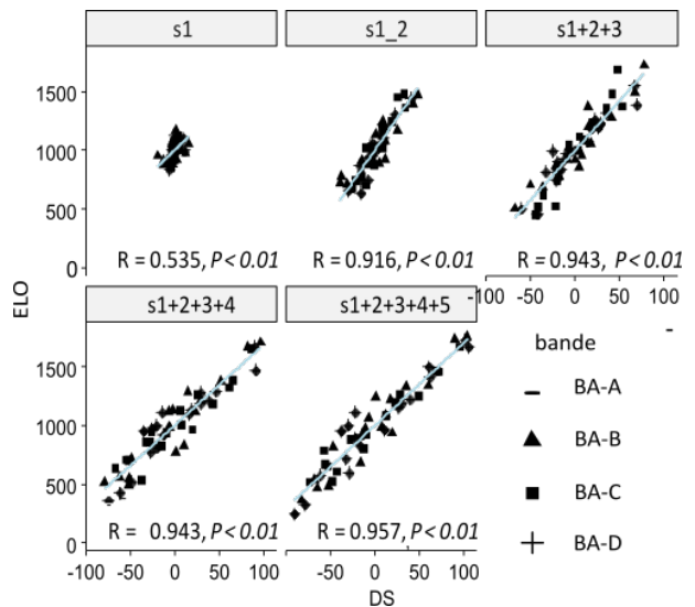
Figure 2 - Corrélation entre elo-score (ELO) et score de David (DS) pour les bandes du protocole A selon les semaines cumulées (R = Coefficient de corrélation de Pearson)
