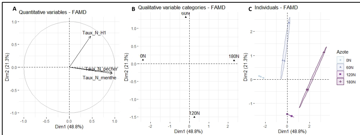
Figure n° 16 : Analyse factorielle de données mixtes réalisée sur les taux d'azote des feuilles de pêcher, de la menthe et du sol entre 0 et 30 cm, correspondant à la période de mi-mai. A : Graphique des variables quantitatives sur les dimensions 1 et 2. B : Graphique de la variable qualitative sur les dimensions 1 et 2. C : Graphique des 12 individus analysés sur les dimensions 1 et 2. Les ellipses représentent les ellipses de confiance autour des points moyens de chaque groupe.
