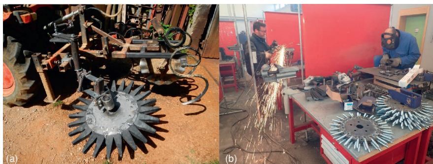
Figure 6.2. Étoile de binage conçue à l'Atelier paysan et qui permet de désherber mécaniquement dans les rangs de vignes ; (a) modèle d'étoile de binage qui s'adapte facilement à différents supports ; (b) les étoiles en cours de fabrication lors d'une formation à l'Atelier paysan (L'Atelier paysan, 2021)
