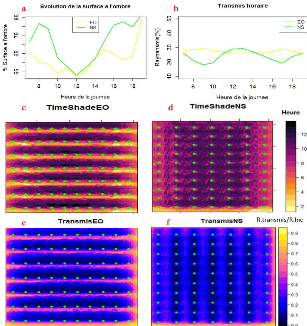
Figure 15 : Comparaison des indicateurs selon l'orientation des rangées d'arbres
