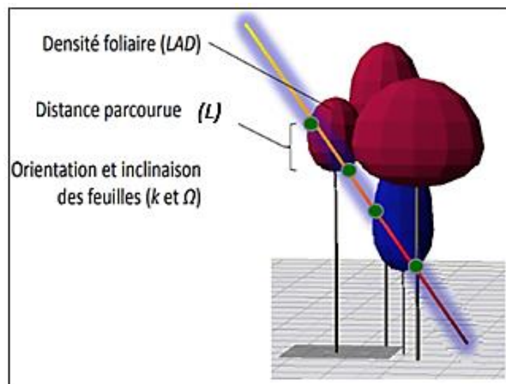
Figure 7 : Interception lumineuse selon l'approche Beer Lambert
