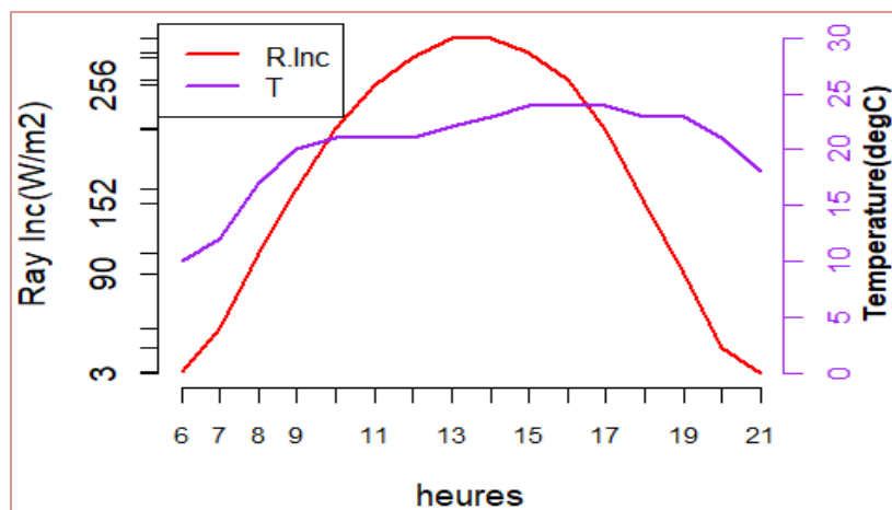
Figure 18 : Rayonnement incident et température sur la station de référence (20/07/2021)
