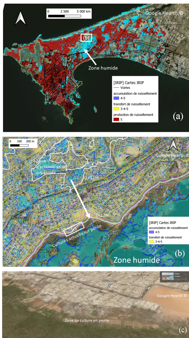
Figure 1. (a, b, c) Localisation des zones de production, transfert-érosion et dépôt-inondation dans la péninsule de Dakar.
