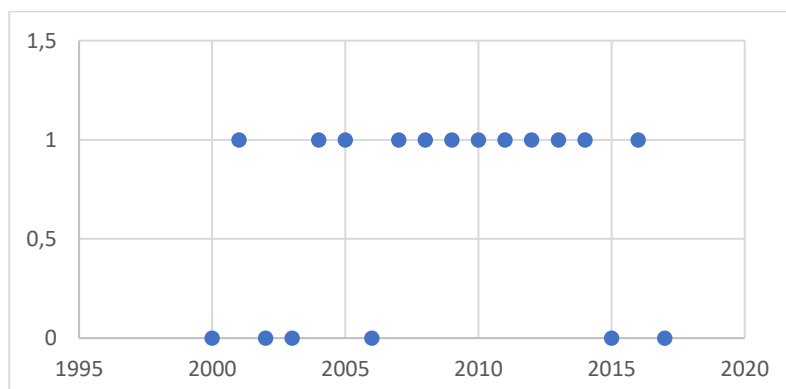
Figure 24 : Présence du test de comparaison des prix
