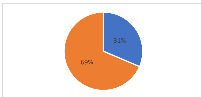
Figure 20 : Taux de remise en cause par la procédure
