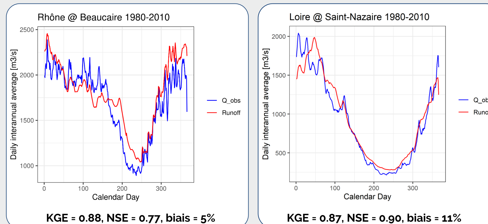
Fig 1 - Régime hydrologique simulé (en rouge) et observé (en bleu) aux exutoires des deux bassins versants.
