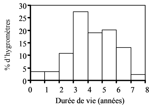
Figure 1 : Proportion d'hygromètres (en %) selon la durée de vie des 84 hygromètres du réseau. Figure 1: Proportion of the 84 hygrometers in the network (in %) according to lifespan.
