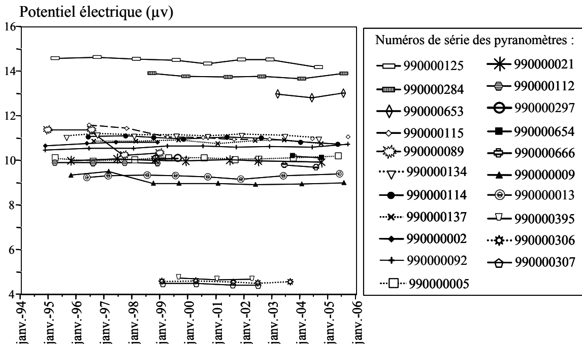
Figure 10 : Variation du potentiel électrique pour chaque pyranomètre, codé par un numéro de série et soumis à un éclairage de 1\text{W/m}^2 , au cours du temps. (Représentation globale des résultats d'étalonnage sans distinguer les dérives des ajustages).
