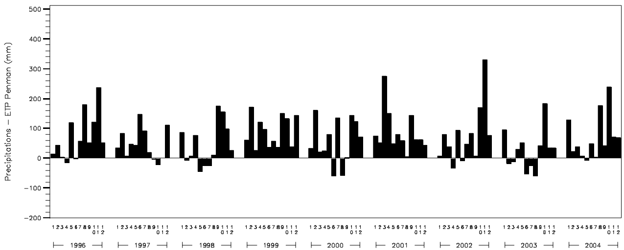
Déficits hydriques mensuels potentiels = (précipitations-ETP Penman)
