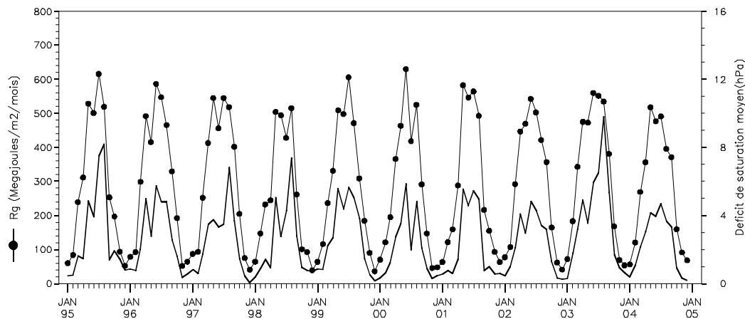
Cumul mensuel du rayonnement global & Moyenne mensuelle du déficit de saturation journalier moyen
