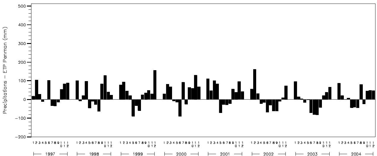
Déficits hydriques mensuels potentiels = (précipitations-ETP Penman)
