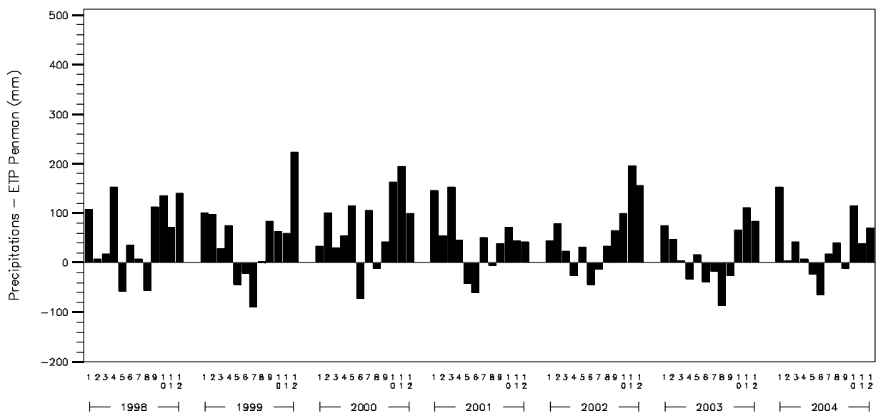
Déficits hydriques mensuels potentiels = (précipitations-ETP Penman)
