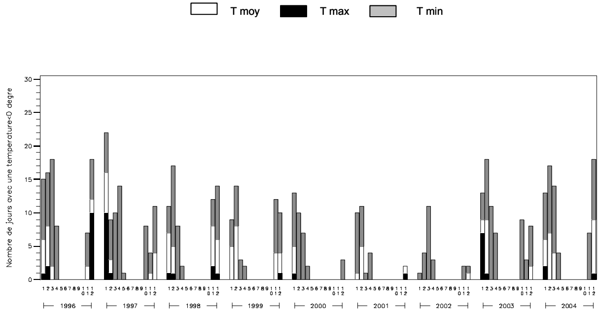
Cumul mensuel des jours caractérisés par une température inférieure à 0°C en considérant les températures journalières moyennes, les minimums et maximums absolus
