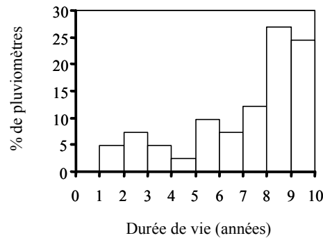
Figure 5 : Proportion des pluviomètres (en %) selon la durée de vie des 41 pluviomètres du réseau. Figure 5: Proportion of the 41 raingauges in the network (in %) according to lifespan.
