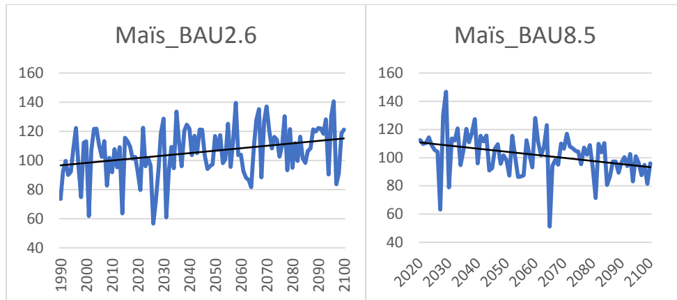
Figure 3 : Simulation par le modèle STICS de la production annuelle de MS du maïs fourrage selon deux scénarios climatiques (RCP2.6 ou RCP8.5), pour le scénario technique Business As Usual ou BAU. Base 100 = production moyenne 1989-2020 de la situation simulée.
