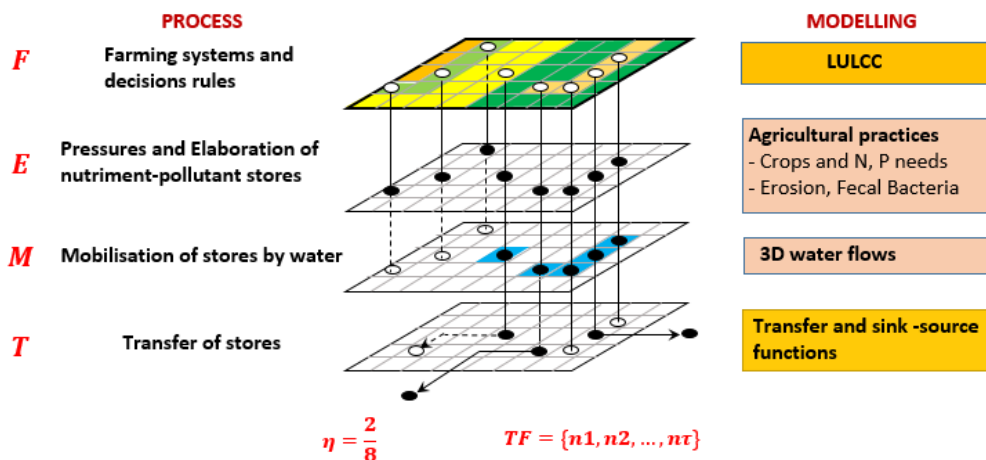
Figure 2 : Schéma d'ensemble des processus et plans de calcul analysés dans OPALÉ. L'espace de calcul est représenté par un domaine maillé formant bassin versant, avec des cellules unitaires de 25m x 25m.
