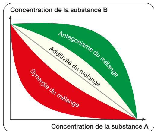
Figure 10. Représentation schématique (isobologramme) des trois types généraux d'interaction entre deux substances A et B. Chaque courbe ou droite représente la combinaison de concentrations de même toxicité (par exemple, la CE50). La droite noire (et son enveloppe blanche) représente l'isobole d'additivité, où l'effet du mélange A + B est égal à celui de la somme des effets individuels de A et de B ; la zone rouge indique une interaction synergique, où l'effet du mélange est plus fort que la somme des effets individuels de A et B ; la zone verte reflète l'antagonisme des deux substances (effet du mélange moins fort qu'attendu sous hypothèse d'additivité).
