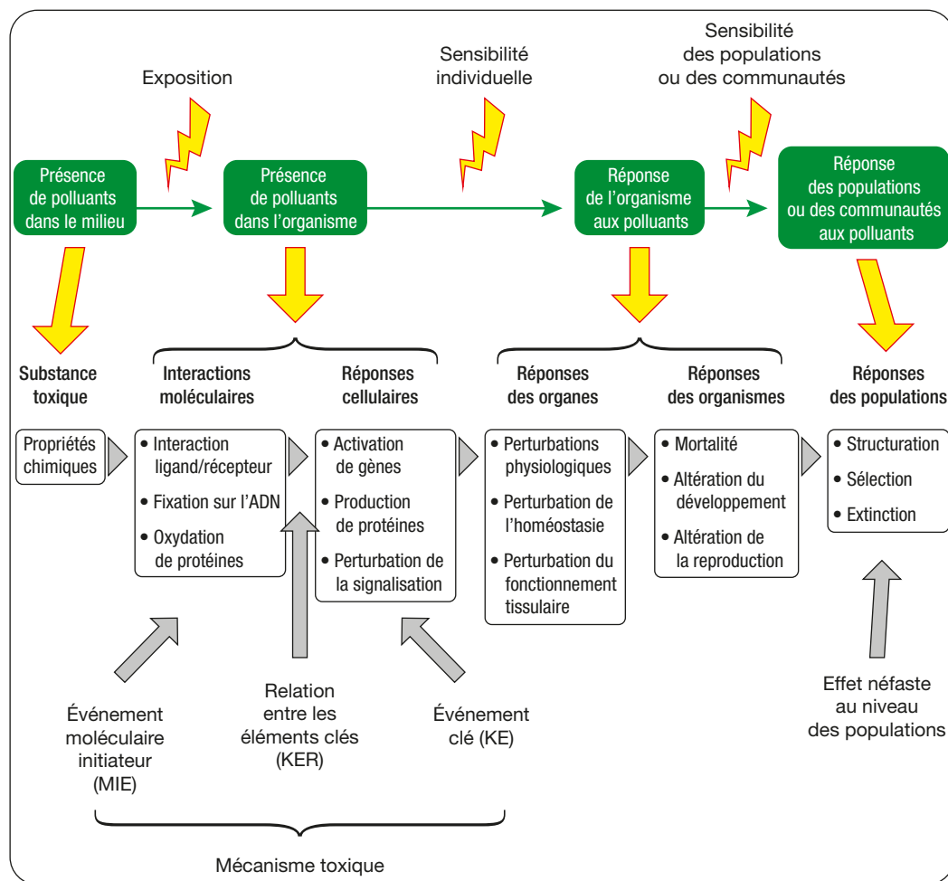
Figure 4. Représentation du cadre conceptuel du chemin de l'effet néfaste ( Adverse Outcome Pathway – AOP) du passage d'un polluant dans un organisme à la suite d'une exposition. Cette exposition se traduit, suivant les sensibilités des organismes, par un effet de la présence du polluant à l'échelle infra-individuelle ou de l'individu, qui se transpose à un niveau biologique supérieur en fonction des sensibilités des populations ou des communautés. Construire une AOP demande à mettre en évidence l'événement initiateur (MIE, Molecular Initiating Event ) et les événements clés (KE, Key Events ) à l'origine des réponses des organismes et des effets sur les populations (d'après Ankley et al. , 2010).
