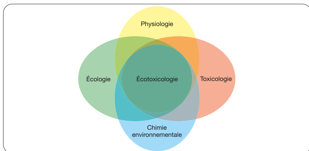
Figure 1. L'écotoxicologie : science intégrative, à l'interface de plusieurs disciplines fondamentales.
