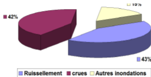
Fig. 1 : Part des inondations par ruissellement dans les inondations déclarées catastrophes naturelles en France (1982-2010) (J. Dehotin, P. Breil, 2011)
