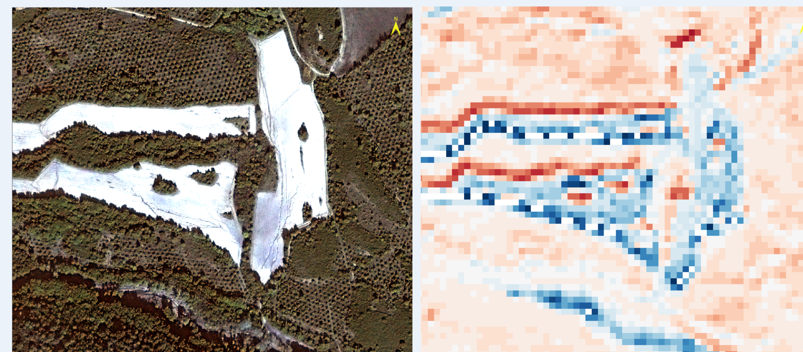
(a) Parcelles affectées par l'aléa érosion. Pléiades: vraies couleurs (b) Sentinel-2: Pente du NDVI (valeurs positives en bleu, négatives en rouge)
