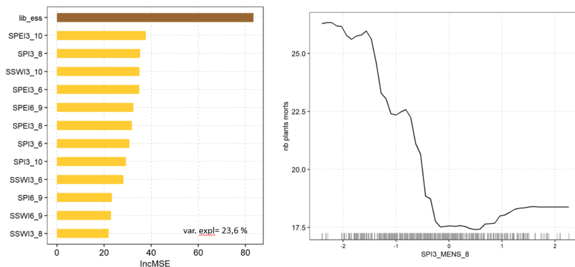
Figure 28 : A gauche, le classement par ordre décroissant d'importance des prédicteurs de la mortalité de plants observée sur le jeu de données des gestionnaires (ONF et GCF), toutes essences confondues. A droite le diagramme de dépendance partielle représentant l'effet marginal de l'indice de sécheresse météorologique (SPI3_8) sur la mortalité des plants. En bas du diagramme, contre l'axe des abscisses, est représentée la distribution du prédicteur.
