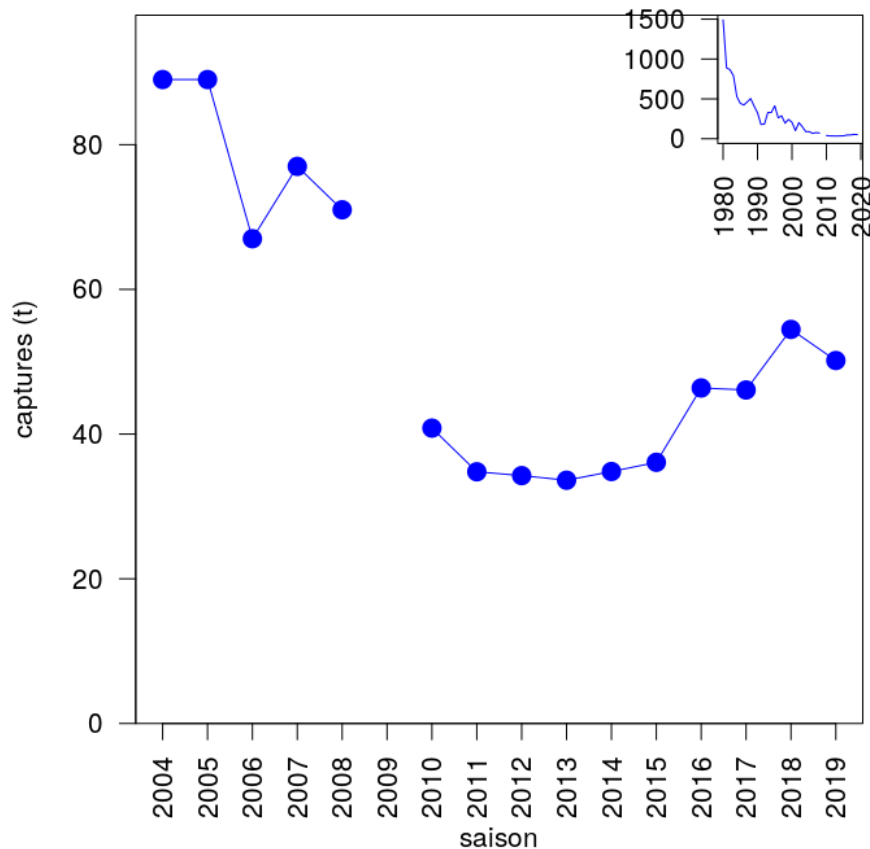
Figure 5 : Captures de 1980 à 2019 (encart en haut à droite), et focus sur le niveau des captures entre 2004 et 2019.
