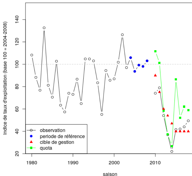
Figure 6 : Évolution de l'indice du taux d'exploitation entre 1980 et 2018 (en base 100 sur la période entre les saisons 2003-2004 et 2007-2008 ; en bleu les valeurs de la période de référence), cibles de gestion (en rouge) et quotas (en vert) retranscrits en taux d'exploitation (voir texte).
