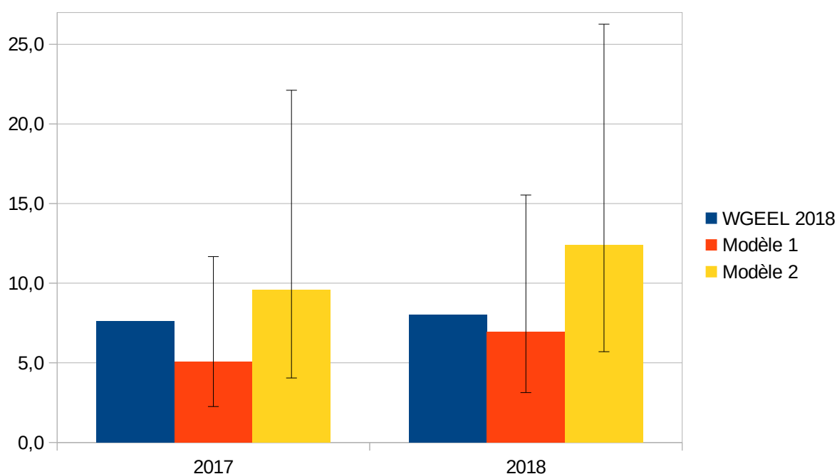
Figure 8 : comparaison entre les résultats des modèles à 1 (modèle 1) et 2 (modèle 2) tendances et la valeur connue aujourd'hui en bleu (ICES, 2018). La barre pour les modèles 1 et 2 correspond à la médiane des distributions a posteriori des prédictions de recrutement tel que donnée dans les rapports d'expertise de chacune des années. Les "moustaches" représentent les intervalles de crédibilité à 95 %.
