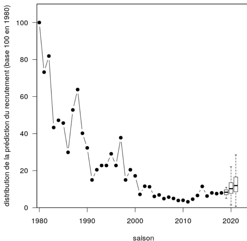
Figure 4 : Évolution du recrutement jusqu'à la saison 2017-2018 (incluse) et distributions des prédictions du recrutement pour les trois saisons suivantes pour le modèle à deux tendances, en incluant les tendances rapportées pour 2018-2019. Les boxplots présentent la médiane, les 1er et 3ème quartiles. Les moustaches correspondent à 1,5 fois l'interquartile.
