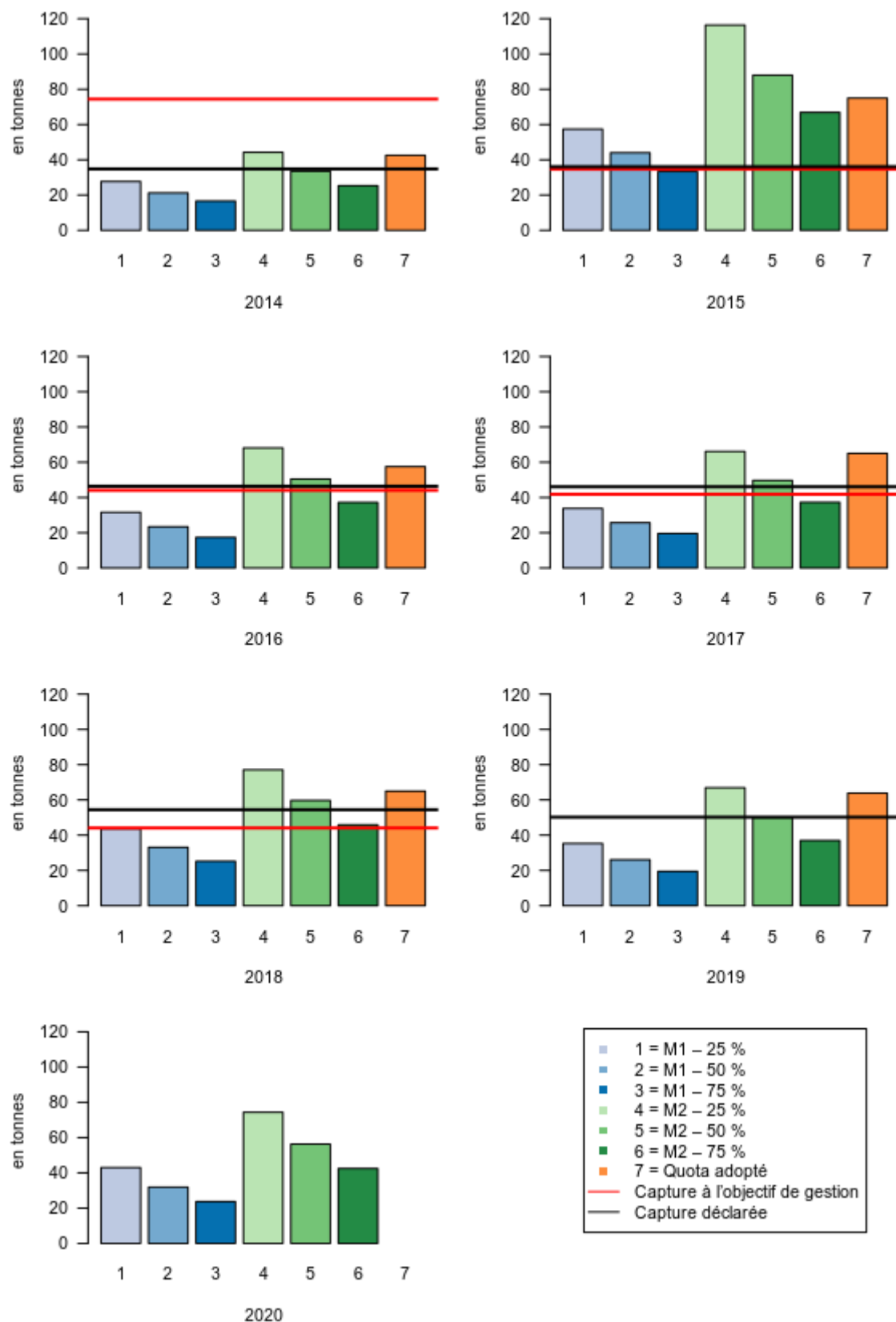
Figure 9 : Comparatif entre les captures déclarées, le quota adopté, la capture maximale respectant à l'objectif de gestion et les TAC calculés chaque année par le CS en fonction du modèle de recrutement (M1 ; M2) et des probabilités d'atteinte de l'objectif (25% ; 50% ; 75%)
