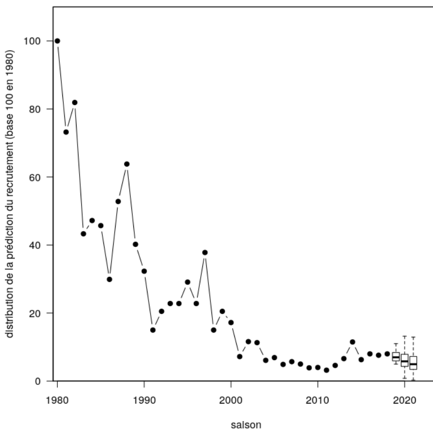
Figure 3 : Évolution du recrutement jusqu'à la saison 2017-2018 (incluse) et distributions des prédictions du recrutement pour les trois saisons suivantes pour le modèle à une tendance exponentielle décroissante, en incluant les tendances rapportées pour 2018-2019. Les boxplots présentent la médiane, les 1er et 3ème quartiles. Les moustaches correspondent à 1,5 fois l'interquartile.
