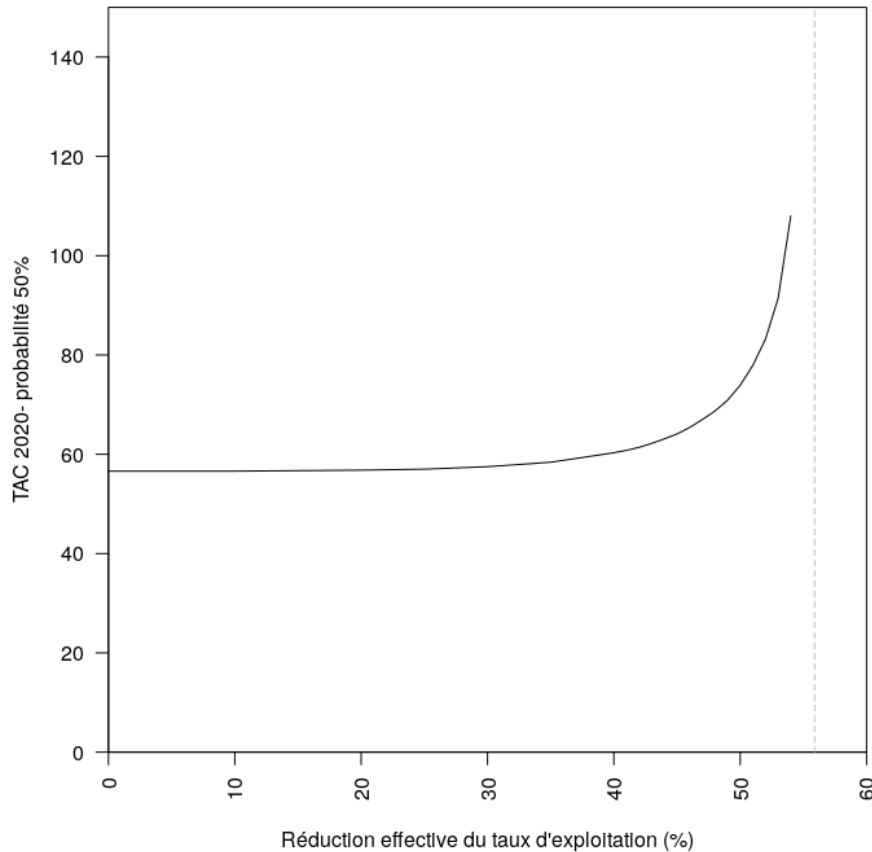
Figure 7 : TAC 2019-2020 estimé en fonction de la réduction effective du taux d'exploitation obtenu avec la diminution du nombre de pêcheurs (ou tout autre mesure) pour le modèle avec changement de régime et une probabilité de 50% d'atteindre la cible de gestion. La ligne verticale en pointillé représente la diminution actuelle du nombre de pêcheur.
