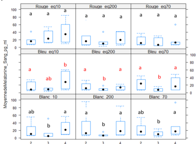
Figure 2 : Valeurs de mélatonine plasmatique (pg/ml) moyennes par modalité d'éclairage entre étapes 2, 3 et 4
