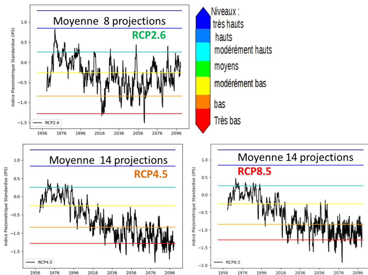
Figure 17 : Evolution moyenne sur le domaine Aqwi-FR et sur l'ensemble des modèles de climat de l'indice piézométrique standardisé de 1950 à 2100 pour les trois scénarios d'émission de gaz à effet de serre.
