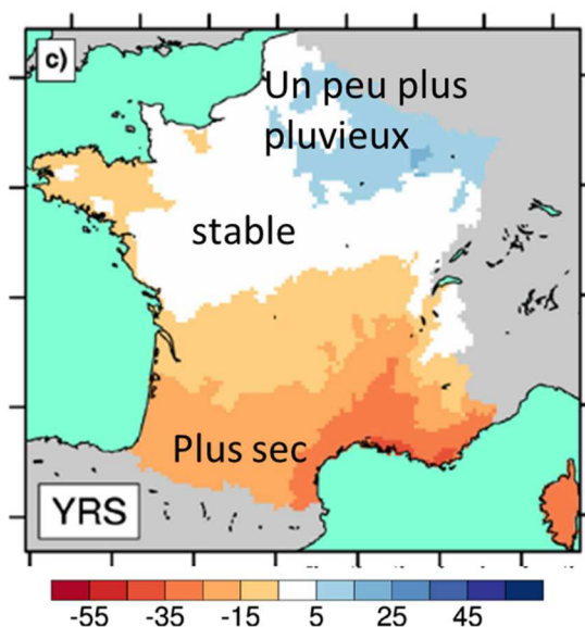
Figure 6 : Evolution en % des précipitations annuelles sur la période 2070–2100 par rapport à la période 1960–1990 en moyenne sur 14 projections climatiques de CMIP5 sous scénarios RCP8.5. Figure issue de Dayon et al. (2018).
