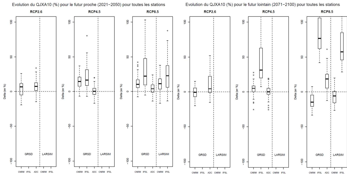
Figure 11 : Idem que la figure précédente pour le débit de crue QJXA10
