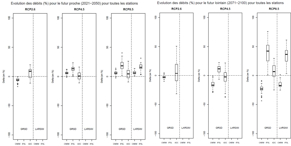
Figure 10 : Distributions des évolutions des débits simulés par deux modèles hydrologiques (GRSD et LARSIM) pour les deux périodes de projection (2021-2050 à gauche ; 2071-2100 à droite) en utilisant trois projections climatiques (CNRM, IPSL et ADC, un ensemble de projections descendues en échelle par la méthode Advanced Delta Change) forcées par trois RCPs 2.6, 4.5 et 8.5, sur l'ensemble des bassins de la zone d'étude. Les évolutions en pourcentage de l'ensemble des stations sont agrégées dans les boîtes à moustaches. A noter que sont absents les scénarios radiatifs RCP 2.6 et 4.5 pour LARSIM ainsi que IPSL RCP 2.6
