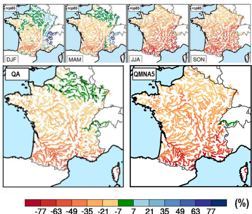
Figure 7 : Moyenne d'ensemble des changements relatifs des débits saisonniers, du module QA et du QMNA5 pour la période 2070-2100 par rapport à la période 1960-1990 pour le RCP 8.5.
