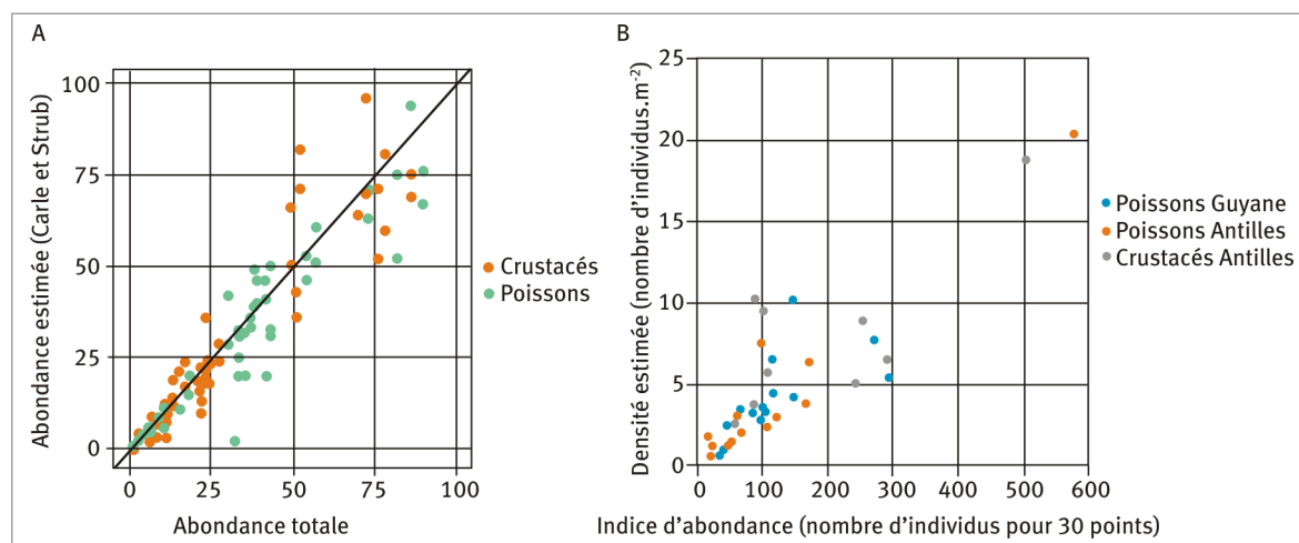
Figure 6 – Relation entre les estimations de densités de poissons et crustacés par enlèvements successifs et A) Les densités vérifiées sur secteurs clos sur des petits cours d'eau des Antilles ; B) Le nombre d'individus capturées pour 30 points d'échantillonnage ponctuel d'abondance (EPA) en Guyane et aux Antilles.
