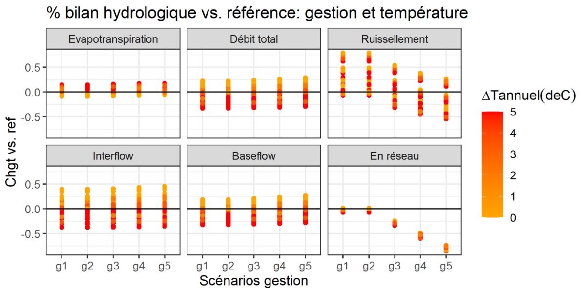
Figure 50 –Evolution de la part de chaque composante du bilan hydrologique annuel (moyenné), par rapport à la simulation de référence, en fonction des scénarios de gestion, et des scénarios de pluie (haut) et de réchauffement (bas)
