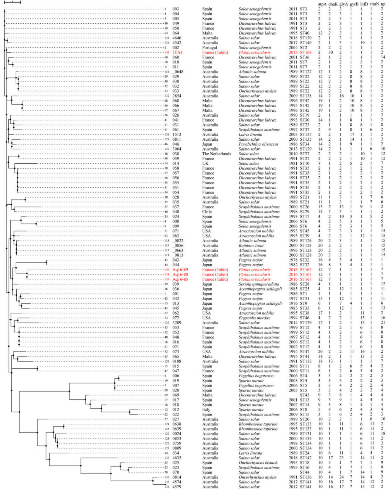
Tree scale: 0.001
