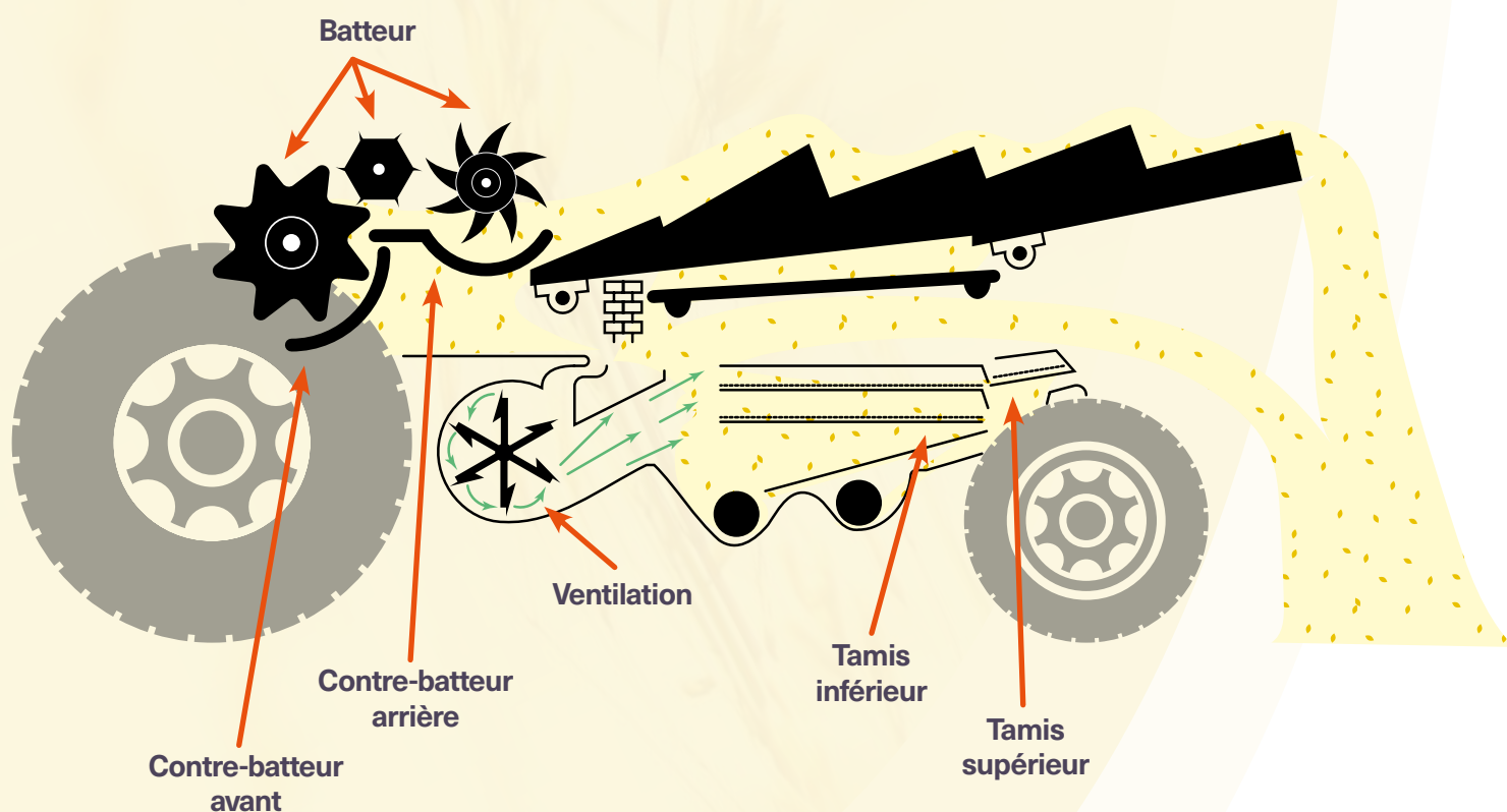
Figure 17 • Schéma de fonctionnement d'une moissonneuse-batteuse (A. Morrison)
