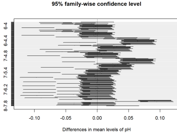
Figure 7 : Résultat méthode de Tukey avec la variable worganic et le site de Laqueuille
