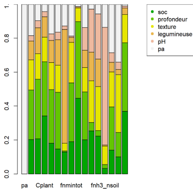
Figure 26 : Diagramme en bâtons de la contribution des entrées sur les sorties (axe des abscisses : pa, gpp, Nplant, Cplant, wshtotsum, yieldnsum, bnfsum, fnmintot, worganic, nn2odenit, fn2osoilatm, n2oemissionsum, fnh3_nsoil, leachsum, n2denitrifsum, RECO)
