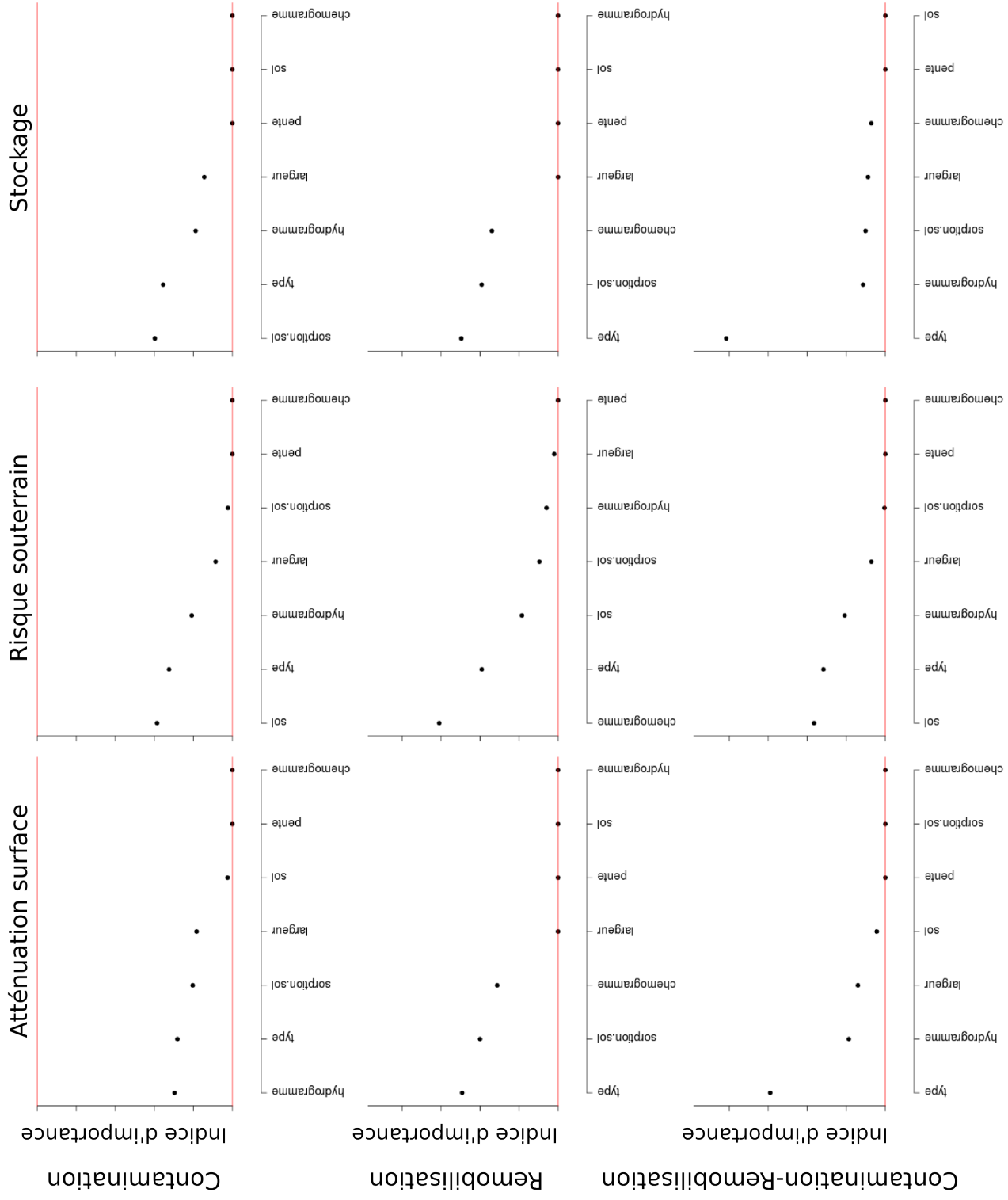
FIGURE E.3 – Indice de sensibilité des facteurs sur les trois indicateurs de contamination (gauche : atténuation de surface, milieu : risque souterrain, droite : stockage) dans le cas d'une contamination par une molécule hydrophobe en Contamination (haut), Remobilisation (milieu) et Contamination-Remobilisation (bas). Plus le facteur est proche de 1 plus le facteur joue sur l'indicateur.
