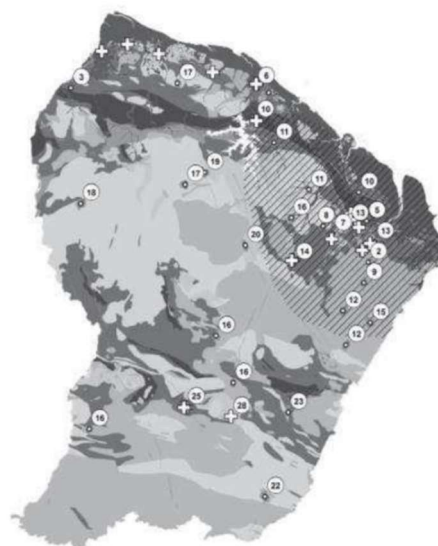
Figure 21 : Carte de répartition des sites de mesure de stock de carbone (Guitet, 2015)
