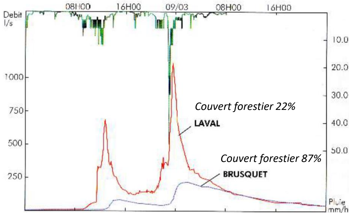
Figure 1. Bassins versants expérimentaux de Draix : crues (débit en l/s, échelle de gauche ; courbes en rouge pour le bassin de Laval et en bleu pour celui du Brusquet) des 8 et 9 mars 1991 en réponse à un épisode pluvieux (pluie en mm/h, échelle de droite, courbe en vert.). Le couvert forestier (pins) des bassins de Laval (86 ha) et du Brusquet (108 ha) est respectivement de 22% et 87% les deux bassins ont le même type de sol. L'érosion annuelle moyenne, rapportée à la surface dénudée est respectivement de 170 tonnes/ha et de 5 tonnes/ha.
