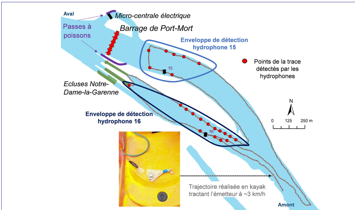
Figure 8. Test de capacité de détection des hydrophones en amont des ouvrages pour évaluer les voies de passage.
