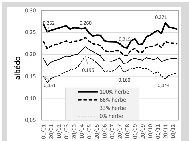
FIGURE 12 : Simulations d'albédo pour différents systèmes d'élevage ; systèmes basés sur un gradient de 100% à 0% d'herbe (100% de cultures) et sol nu Figure 12: Albedo simulations for different livestock systems; systems based on a gradient from 100% to 0% grass (100% crops) and bare soil
