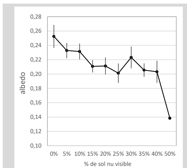
FIGURE 9 : Valeur moyenne (et écart-type) d'albédo du sol des fermes expérimentales, selon la proportion de sol nu visible
