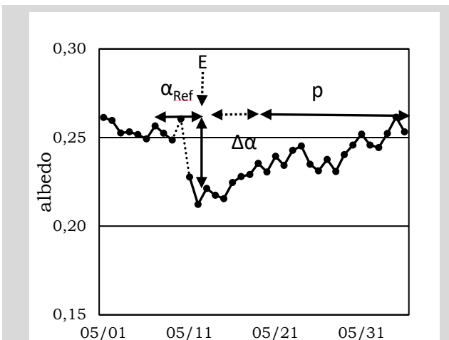
FIGURE 3 : Estimation d'une variation d' \alpha , à la suite d'un évènement (E). Figure 3 : Estimation of a variation of \alpha , following an event (E).
