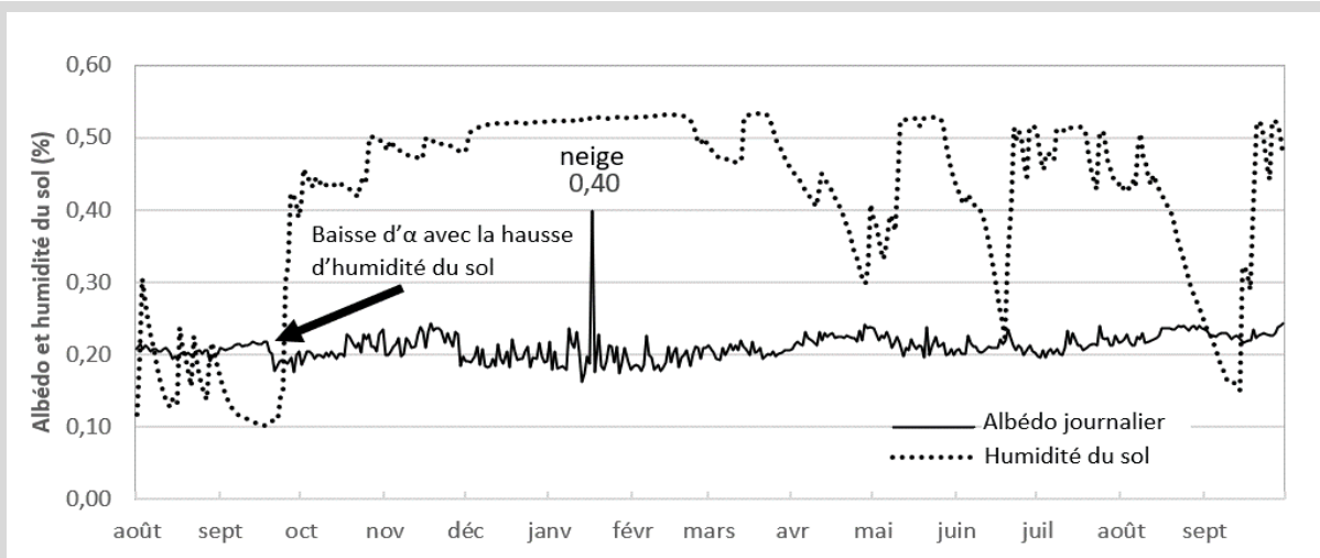
FIGURE 8 : Albédo moyen quotidien et d'humidité du sol sur le site de Jalogny. Figure 8 : Average daily albedo and soil moisture at the Jalogny site.
