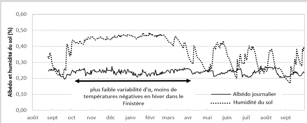
FIGURE 7 : Albédo moyen quotidien et d'humidité du sol sur le site de Trévarez. Figure 7 : Average daily albedo and soil moisture at the Trévarez site.
