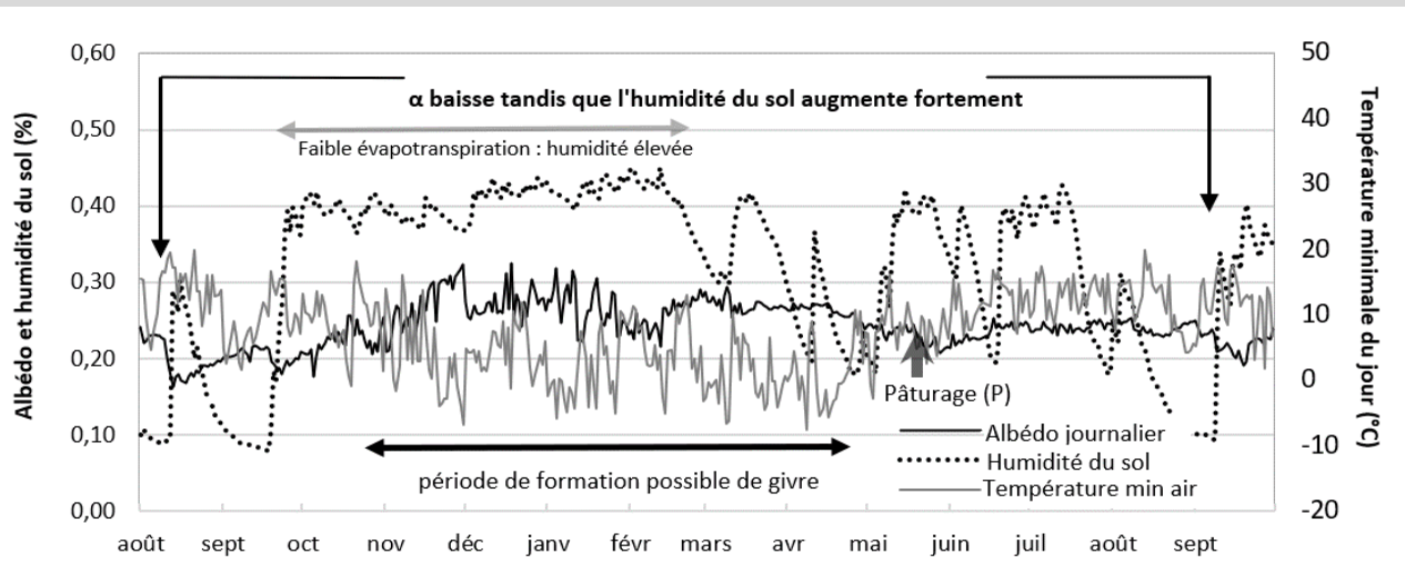
FIGURE 6 : Dynamique d'albédo et d'humidité du sol et des températures minimales sur le site du Mourier. (min = minimale). Figure 6 : Dynamics of albedo and soil moisture and minimum temperatures at the Mourier site. (min = minimum).
