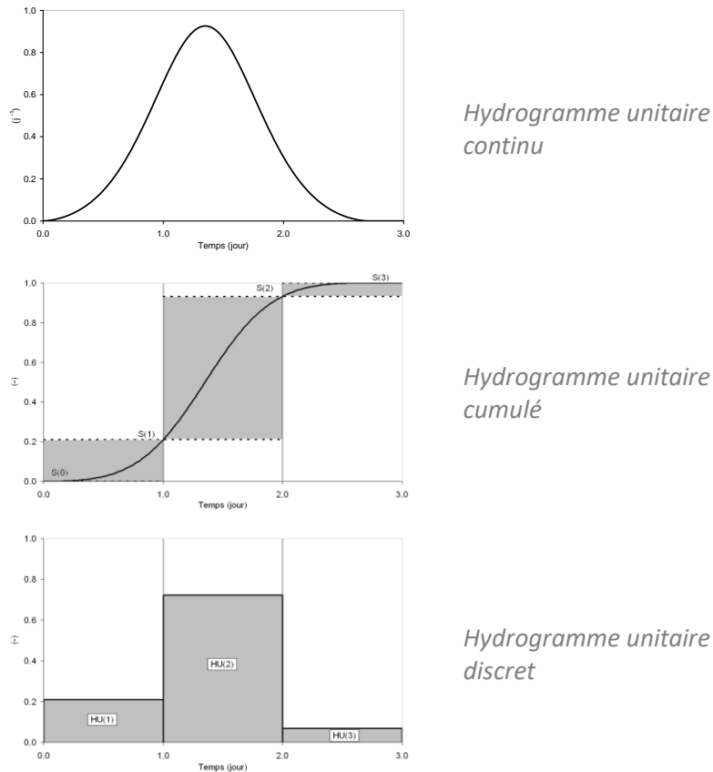
Figure 23 : De l'hydrogramme continu à l'hydrogramme discret
