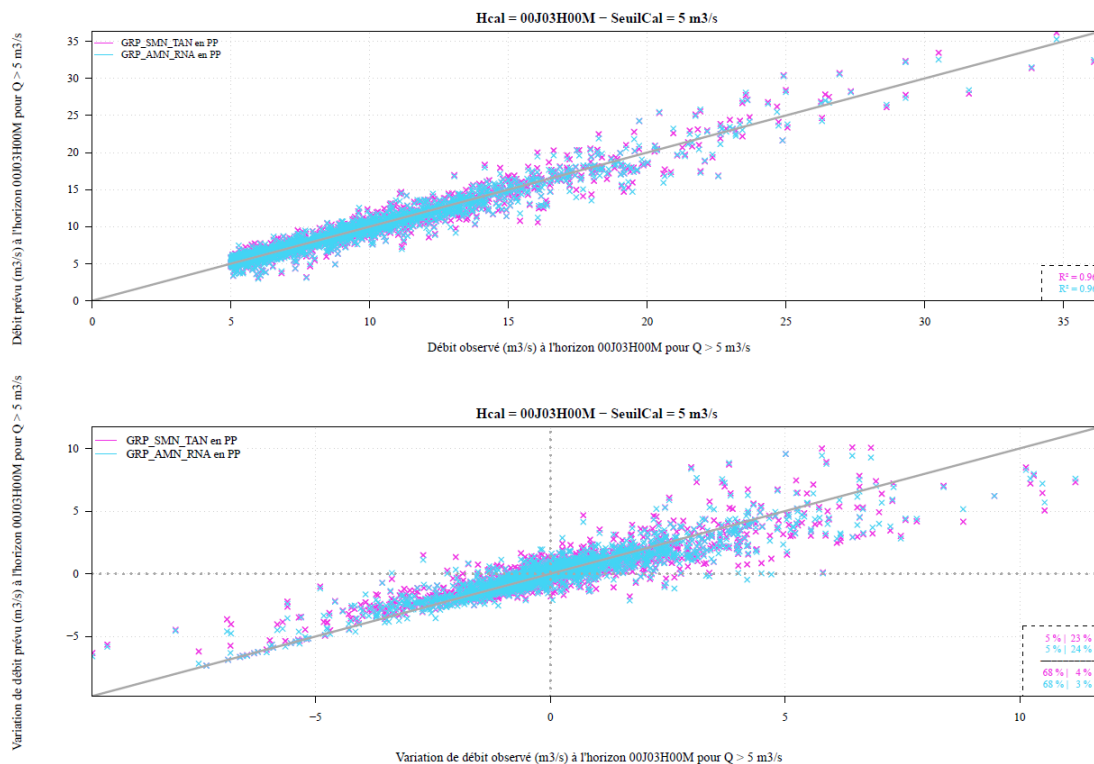
Figure 14 : Exemple de fiche synthétique des résultats
