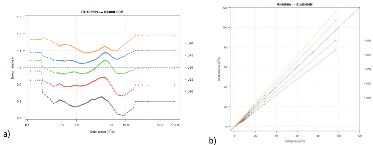
Figure 16 : Résultats du calage des abaques d'incertitudes prédictives a) quantiles d'erreur relative pour les 101 points de référence, b) quantiles de la distribution des valeurs que peut prendre le débit observé pour les 101 points de référence de débits prévus
