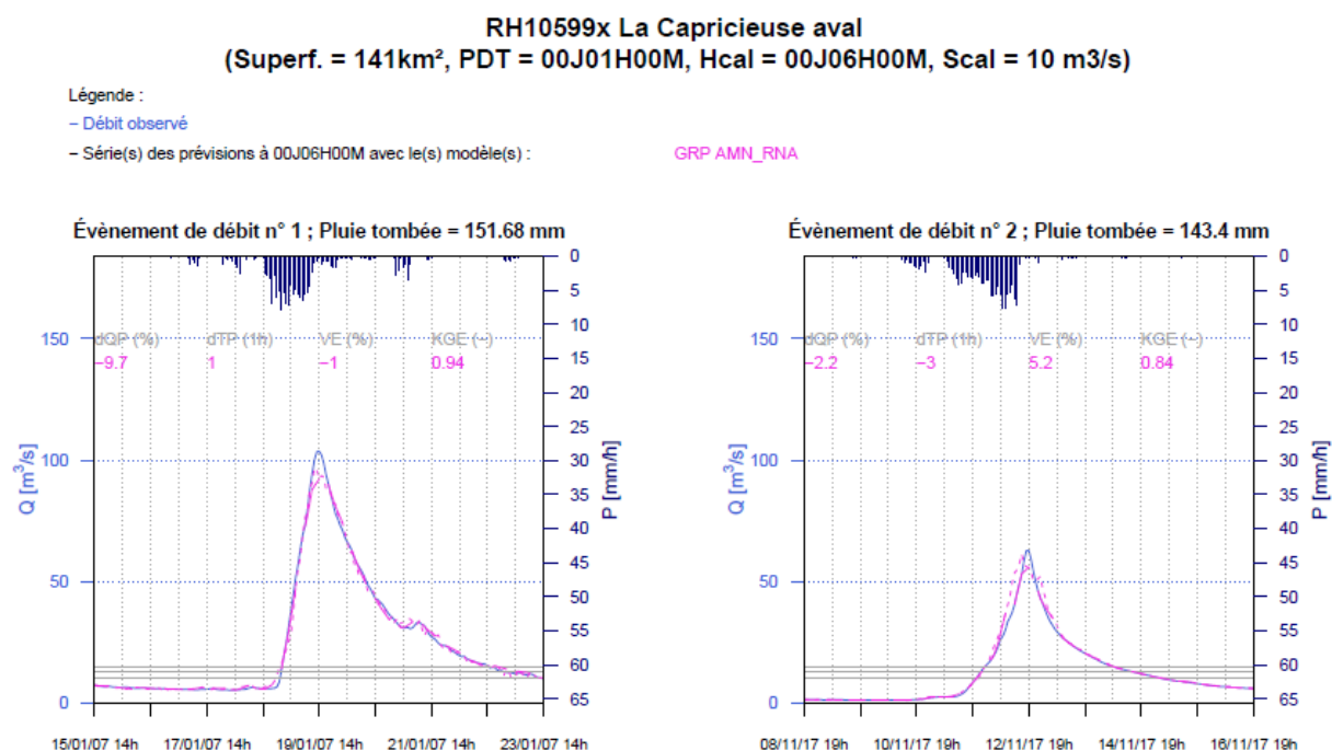
Figure 15 : Exemple de représentation des résultats du modèle sur des événements sélectionnés
